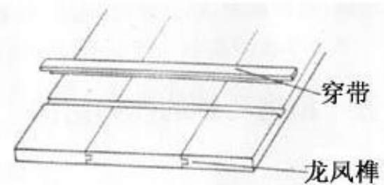
龙凤榫加穿带
