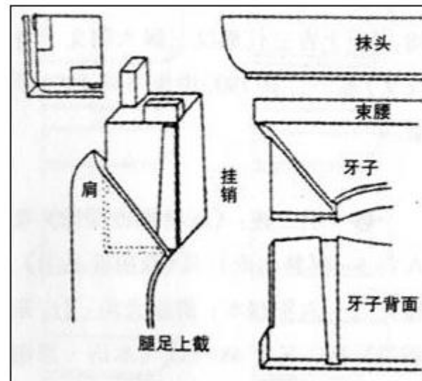
抱肩榫
