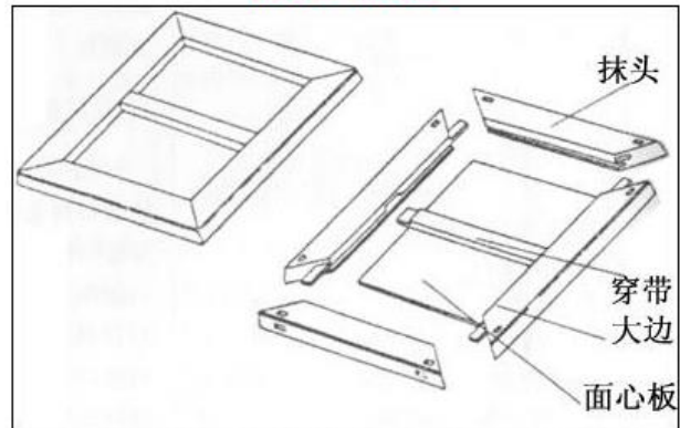
攒边打槽装板
