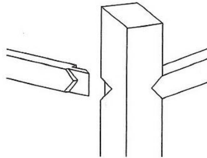
平尖肩榫结构
