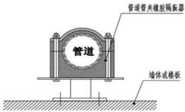
管道落地支撑隔振处理图
