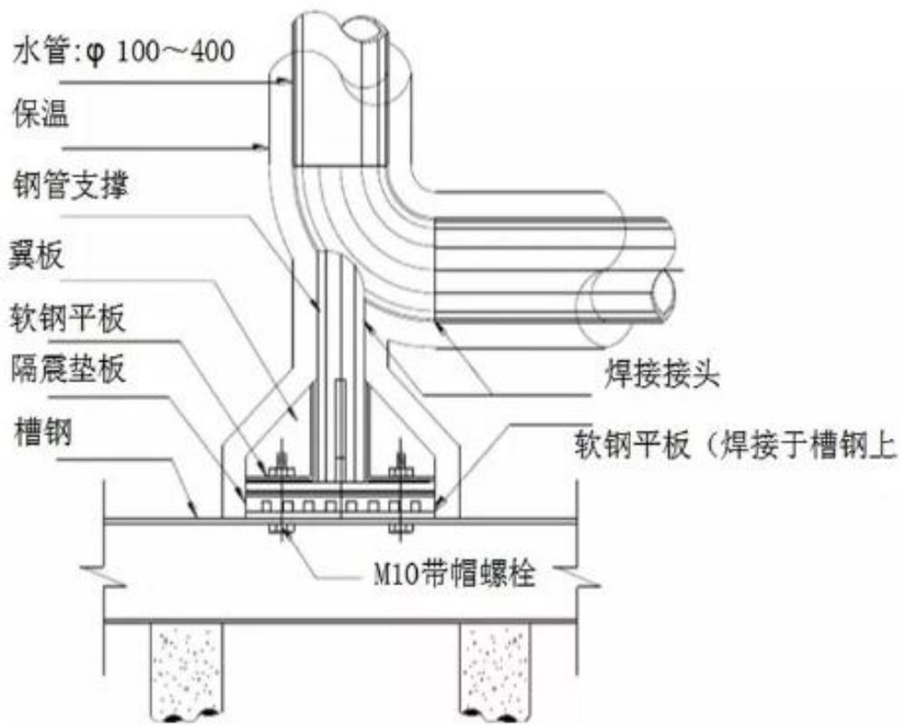
管道消声处理
