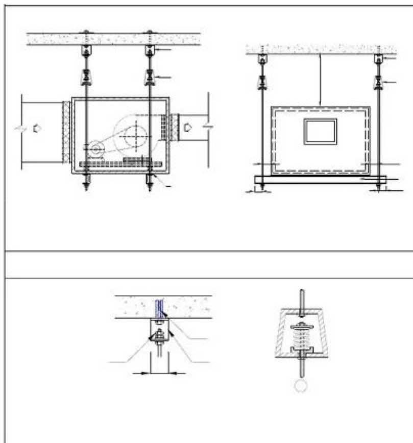
轴流风机防振吊钩
