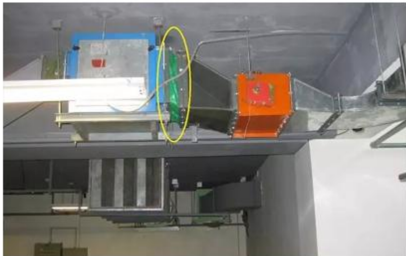
防水帆布接头
