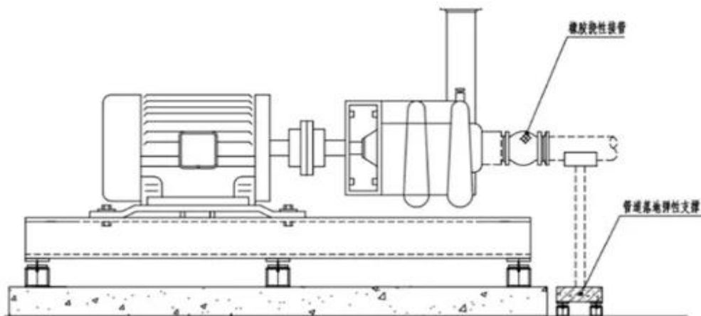
卧式水泵隔振处理图
