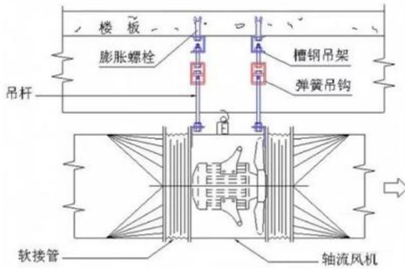
阻尼弹簧减震器
