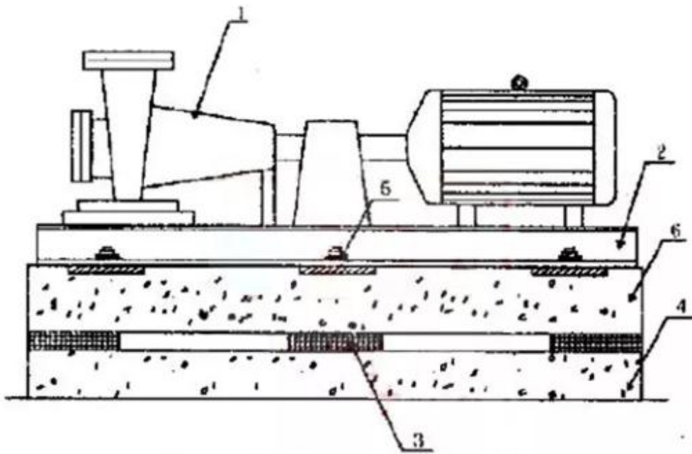
1. 水泵；2. 水泵自带槽钢支架；3. 橡胶减震垫；4. 水泵基础（高度>50nm）；5. 预埋钢板；6. 混凝土减振台座。 水泵减震台座减震形式
