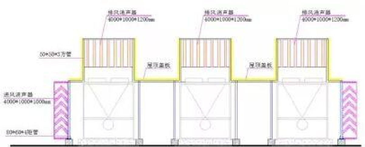
中央空调外机降噪
