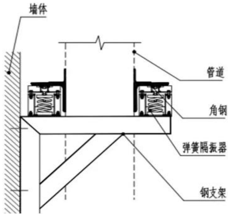
管道落地支撑支架减振处理
