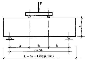
图 10.0.3 抗折试验装置
