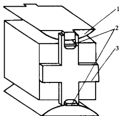
图 4.5.3 支架示意
