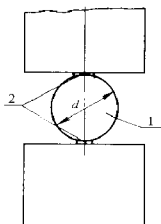
图 D.0.4-1 劈裂抗拉试验
