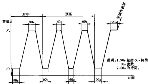
图 8.0.4 弹性模量加荷方法示意图
