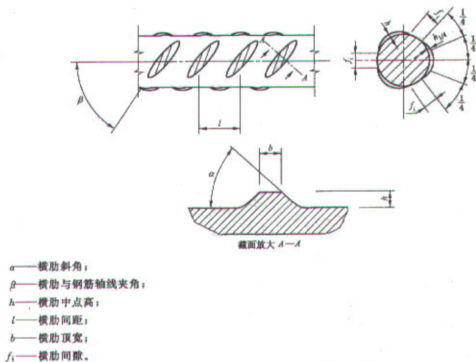
图1 三面肋钢筋表面及截面形状
