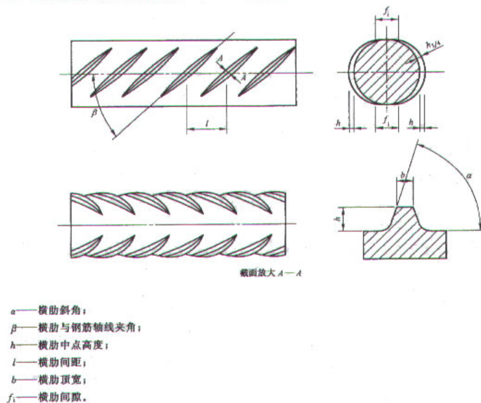
图2 二面肋钢筋表面及截面形状
