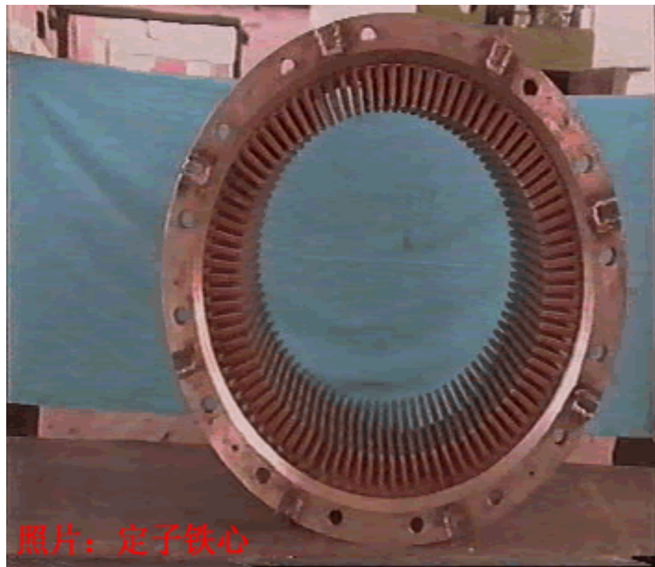
照片：定子铁心
