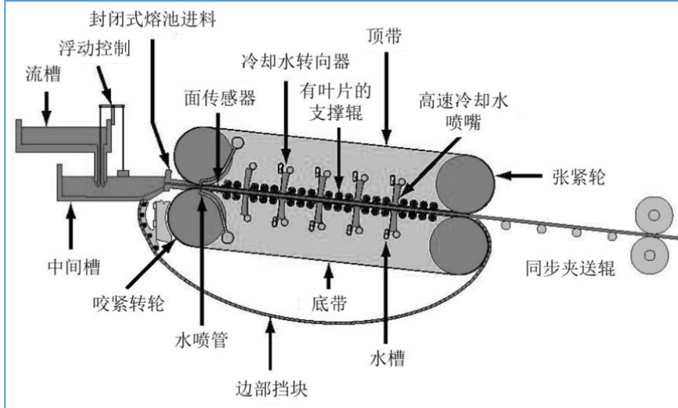
Hazelett 双带连铸机原理图
