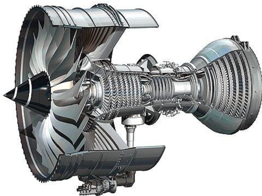
航空发动机
