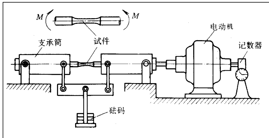
疲劳实验机
