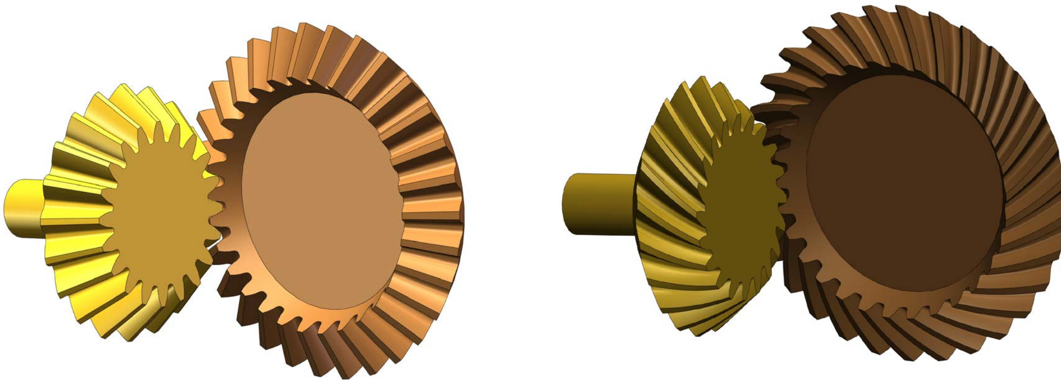
锥齿轮传动
