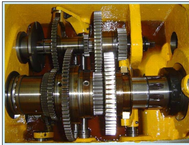
机床主轴箱
