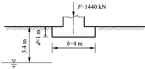
(a) 地基与基础剖面
