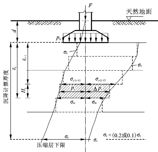
图 2-25 分层总和法计算地基最终沉降量
