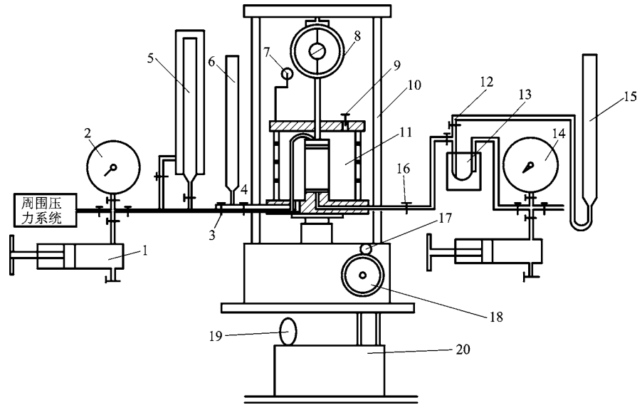
1—调压筒; 2—周围压力表; 3—周围压力阀; 4—排水阀; 5—体变管; 6—排水管; 7—变形量表; 8—量力环; 9—排气孔; 10—轴向加压设备; 11—压力室; 12—量管阀; 13—零位指示器; 14—孔隙压力表; 15—量管; 16—孔隙压力阀; 17—离合器; 18—手轮; 19—马达; 20—变速箱。
