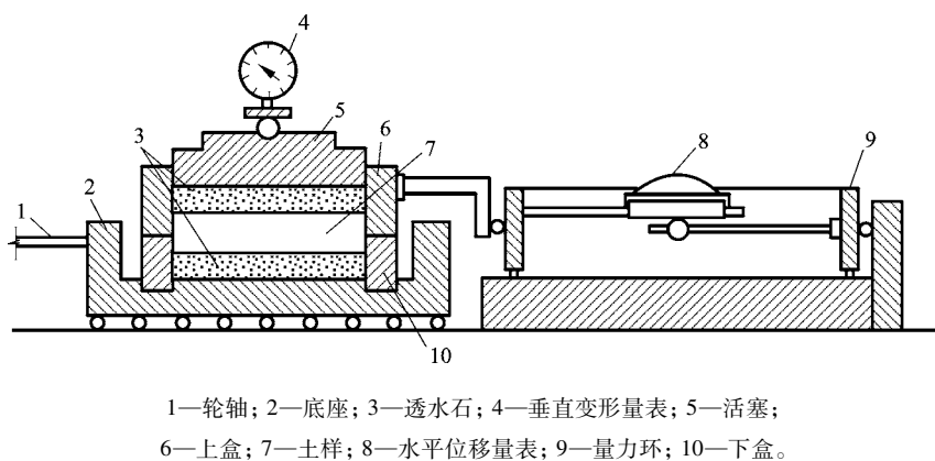
图3-8 应变控制式直剪仪
