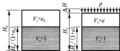
图 2-21 土样侧限压缩孔隙体积变化示意图
