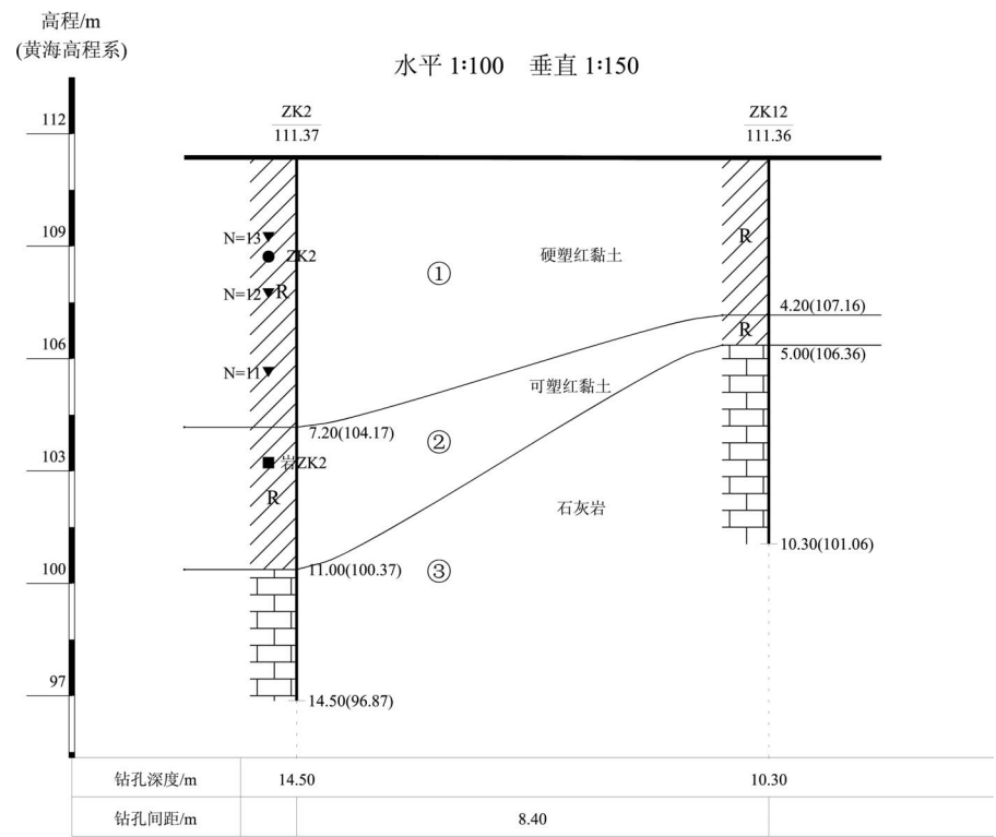
(c)地质剖面图 8—8′
