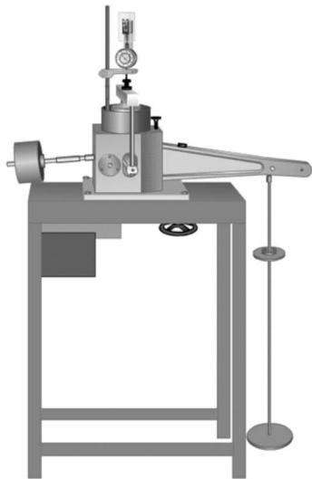
图 2-34 固结仪
