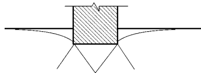
图3-19 冲切破坏
