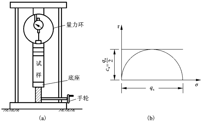
图 3-12 无侧限试验极限应力圆
