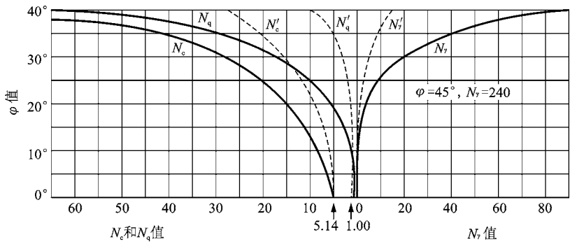
图 3-23 太沙基极限承载力系数图
