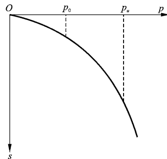
图 2-24 现场载荷试验 p-s 曲线
