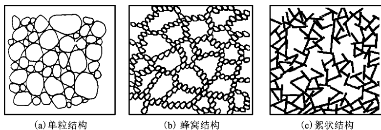
图 1-8 土的结构示意图
