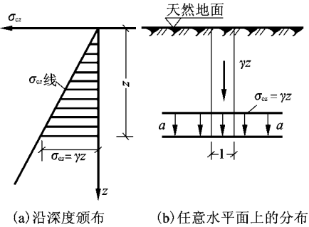
图 2-1 均质土中竖向自重应力
