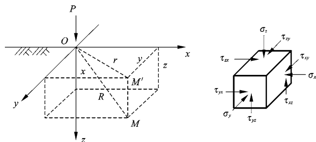
图 2-10 集中力作用下地基中 M 点的应力状态
