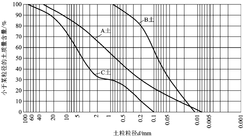
图 1-9 三种土样 A、B、C 的颗粒级配曲线
