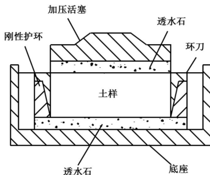
图 2-20 土的压缩仪构造示意
