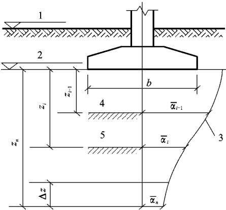
1—天然地面标高；2—基底标高；3—平均附加应力系数 \bar{\alpha} 曲线；4— i-1 层；5— i 层。
