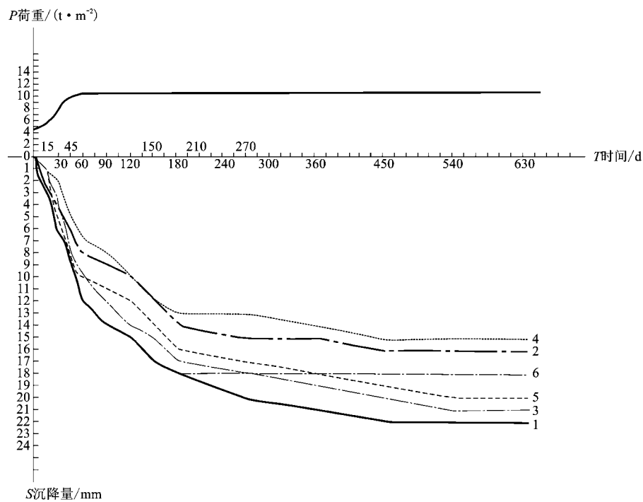
图 2-33 某建筑物时间 - 荷载 - 沉降量曲线图
