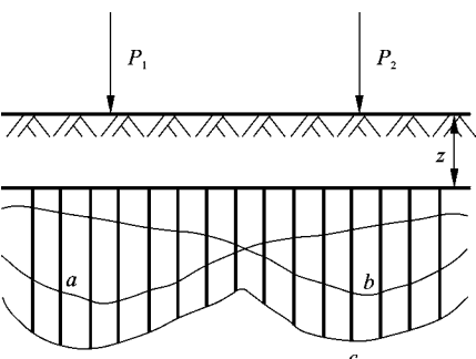
图 2-13 两个竖向集中力作用下地基附加应力 \sigma_z 的叠加
