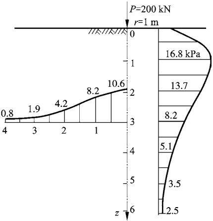
图 2-14 附加应力分布结果
