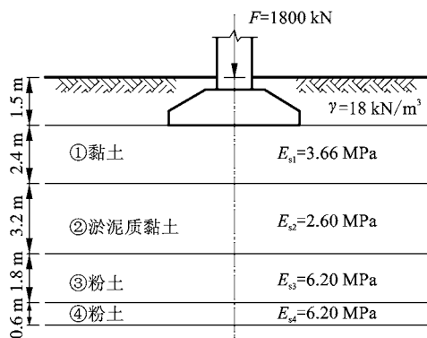
图 2-28 例题 2-7 的地基与基础剖面示意
