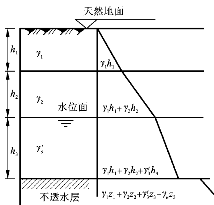
图 2-4 层状分布地基土的自重应力
