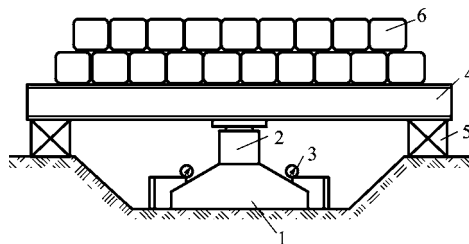
1—承压板; 2—千斤顶; 3—百分表; 4—平台; 5—枕木; 6—堆重。
