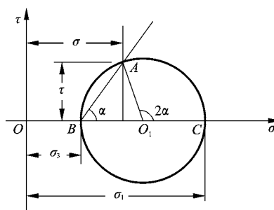
图 3-3 用莫尔应力圆求正应力和剪应力
