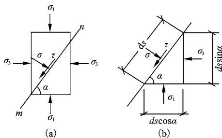
图 3-2 土中任一点的应力
