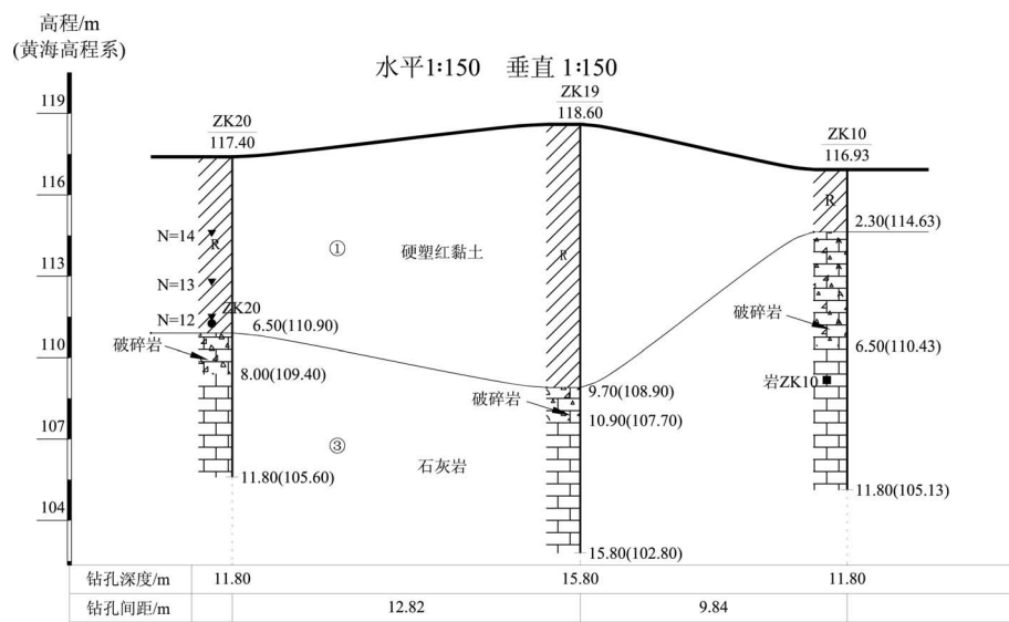
(b)地质剖面图 5—5′
