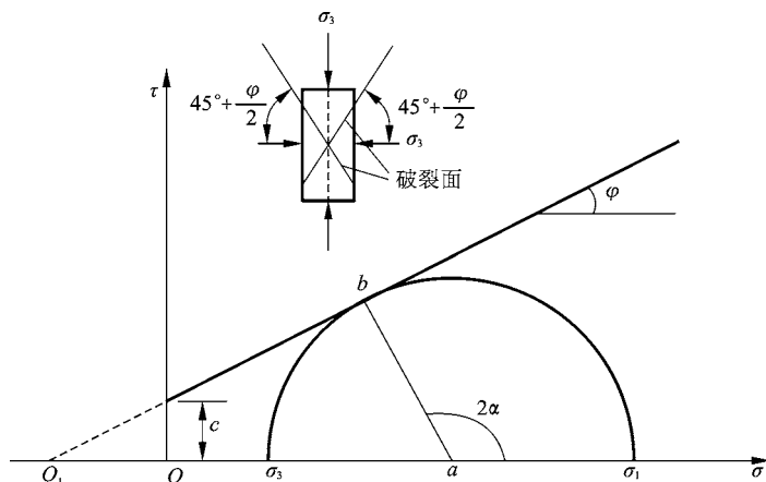
图 3-7 土的破裂面确定
