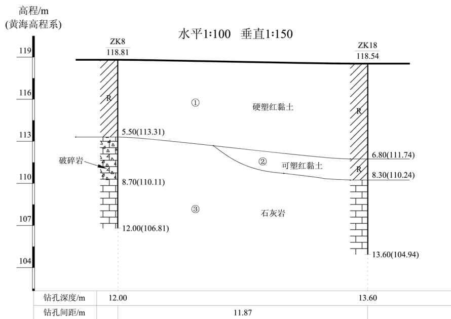
(e)地质剖面图 14—14′
