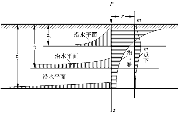
图 2-11 地基附加应力 \sigma_z 的分布规律
