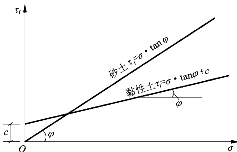
图3-1 砂土与黏性土的抗剪强度 \tau_f 与法向应力 \sigma 的关系曲线
