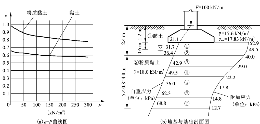
图 2-26 例题 2-6 的示意图
