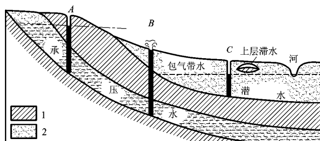
图 1-6 地下水埋藏示意图
