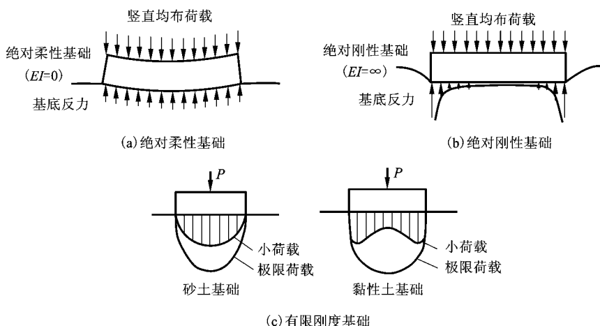
图 2-5 地基与基础的相对刚度对基底压力分布的影响
