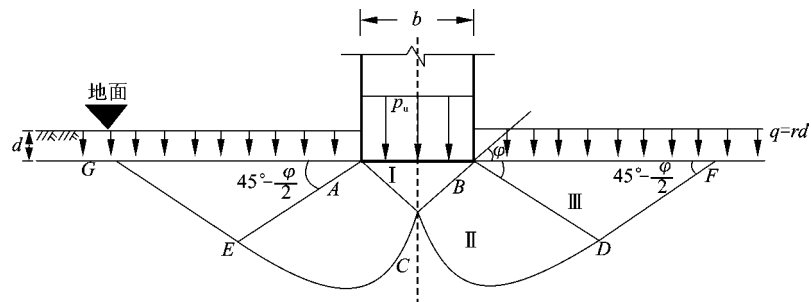
图 3-22 条形均布荷载作用下太沙基公式地基滑动面形状
