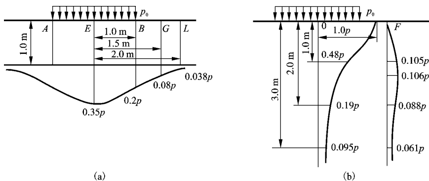
图 2-19 例题 2-4 中的地基附加应力扩散规律
