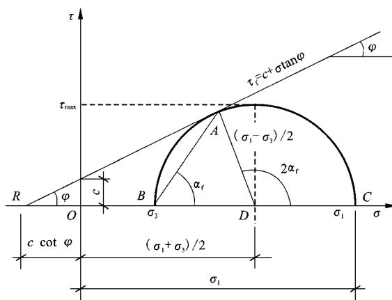
图 3-6 黏性土极限平衡条件示意图
