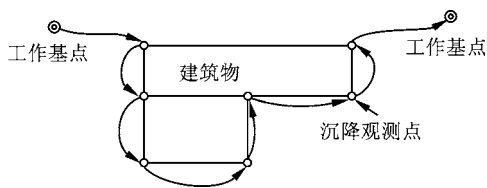
图 2-31 沉降观测方法示意
