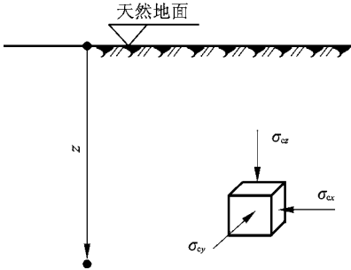
图 2-2 地基土中侧向自重应力 \sigma_{cx} 和 \sigma_{cy}
