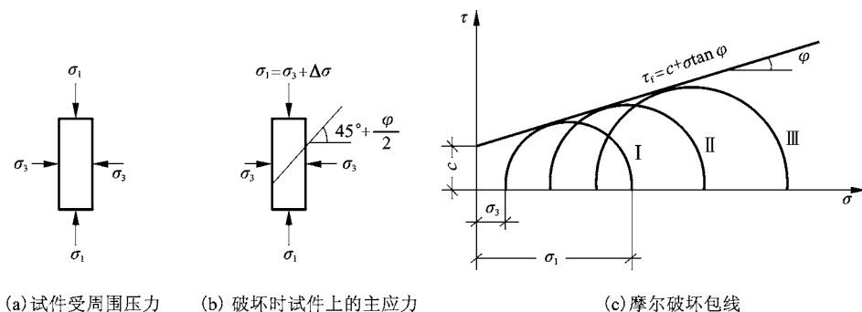
图 3-11 三轴压缩试验原理
