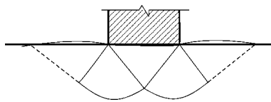
图3-18 局部剪切破坏
