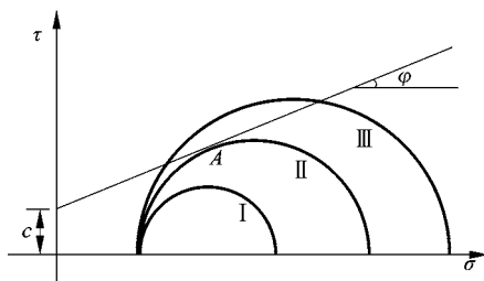
图 3-5 莫尔应力圆与土的抗剪强度之间的关系
