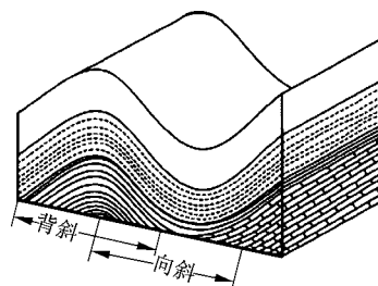
图 1-4 背斜和向斜
