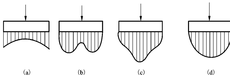
图 2-6 荷载对基底压力的影响
