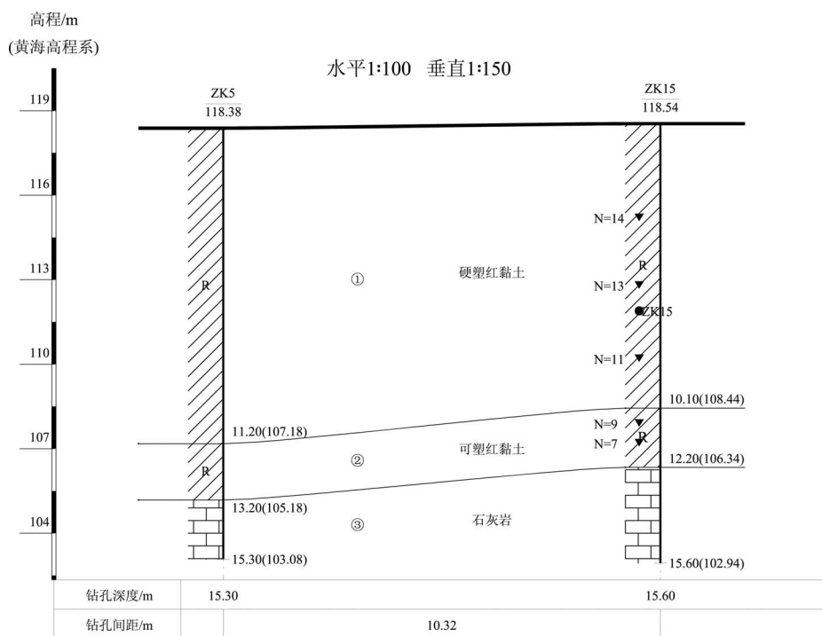
(d)地质剖面图 11—11′
