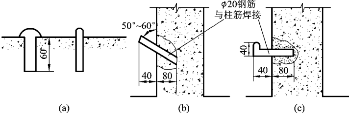
图 2-30 几种沉降观测标志示意
