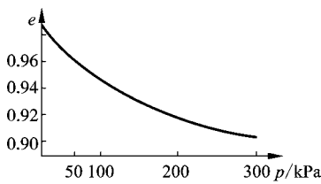
(b) 压缩曲线
