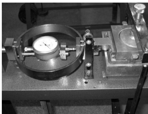
图3-15 测力环细部
