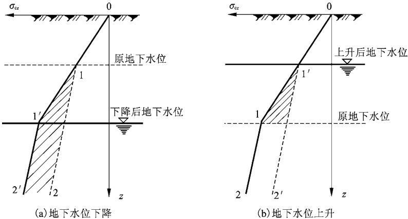
图 2-3 地下水位升降对自重应力的影响
