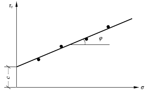
图 3-9 \tau_f - \sigma 关系曲线
