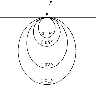
图 2-12 地基附加应力 \sigma_z 的等值线
