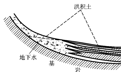
图 1-3 洪积土示意图
