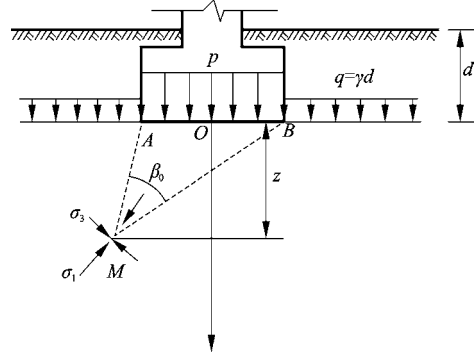
图 3-21 条形均布荷载作用下地基中的主应力
