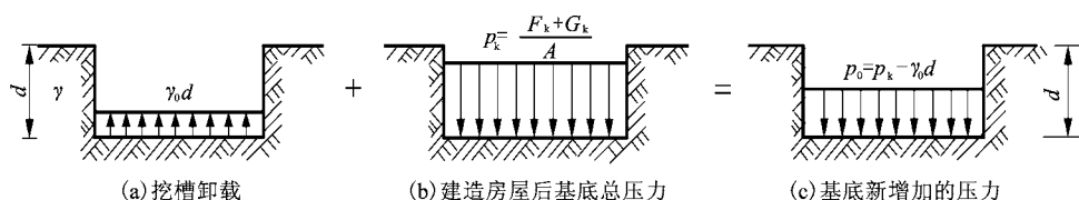
图 2-9 基底附加压力
