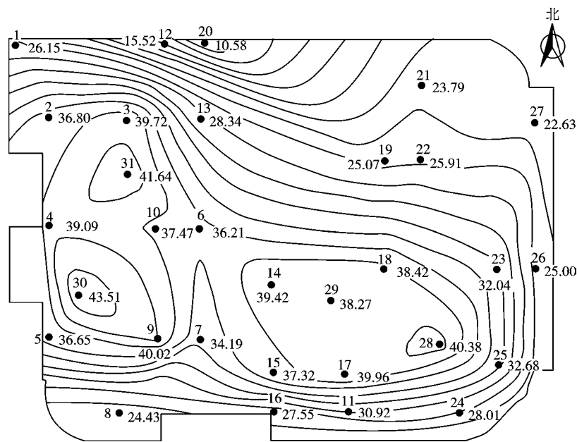
图 2-32 某建筑等沉降曲线图
