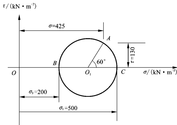
图 3-4 莫尔应力圆
