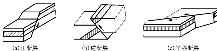
图 1-5 断层
