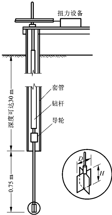
图 3-13 十字板剪切仪示意图
