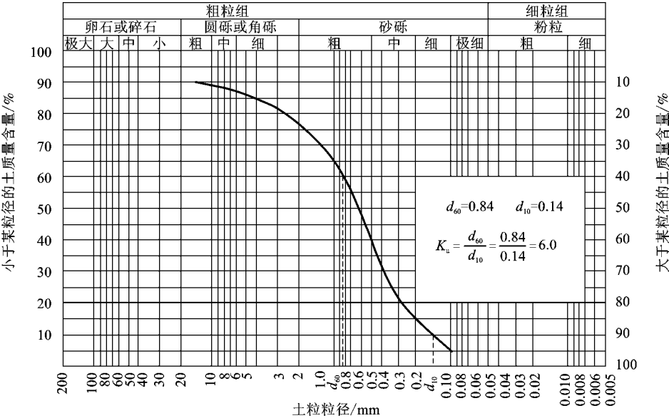
图 1-7 土的颗粒级配累计曲线
