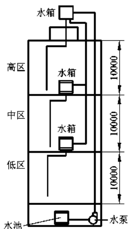
图 2-11 减压水箱给水方式
