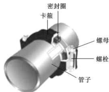
图 2-26 沟槽连接
