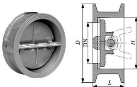
图 2-35 蝶式止回阀
