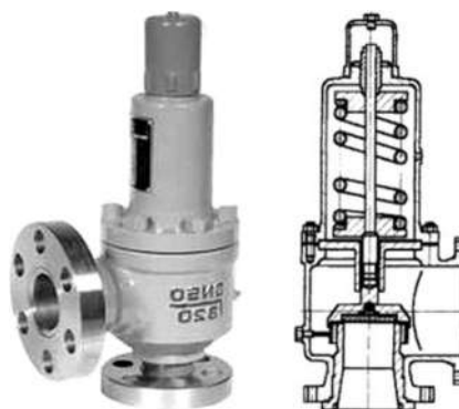
图 2-36 安全阀
