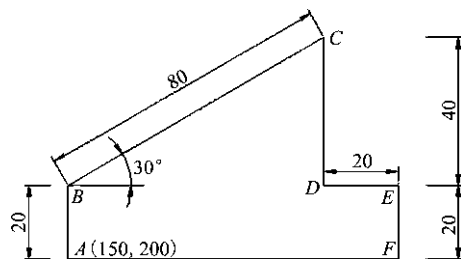
图 1-13 坐标输入实例
