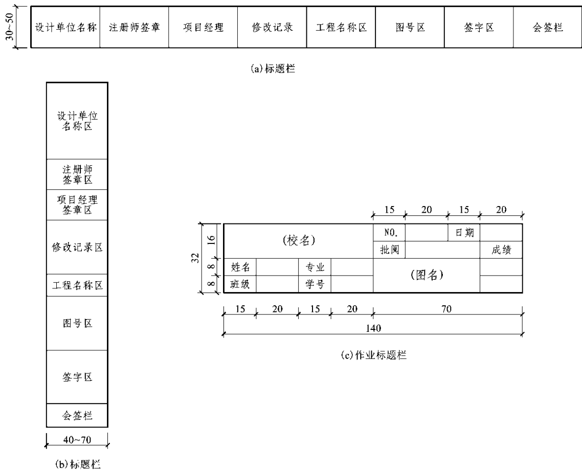
图 2-2 标题栏格式
