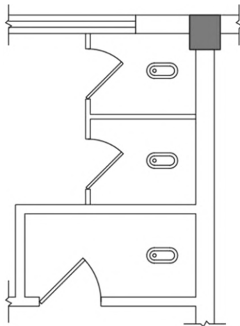
图 3-54 蹲便器
