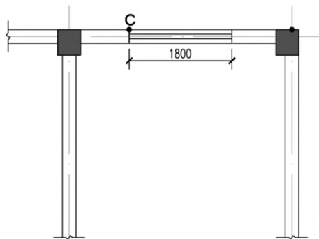
图 3-44 插入的 C-1
