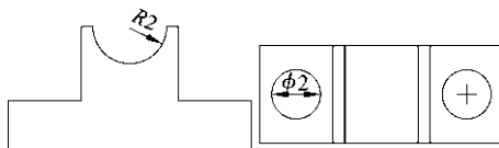
图 1-110 半径、直径与圆心标注
