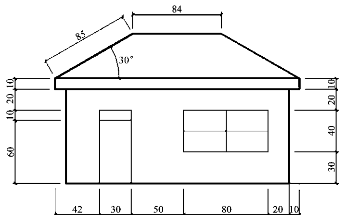
图 1-26 平房立面图
