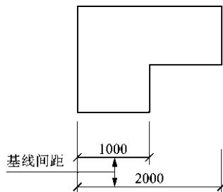
图 1-114 “基线间距”位置示意
