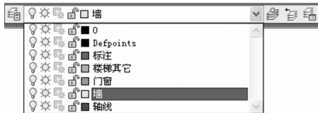
图 1-73 “图层”工具栏
