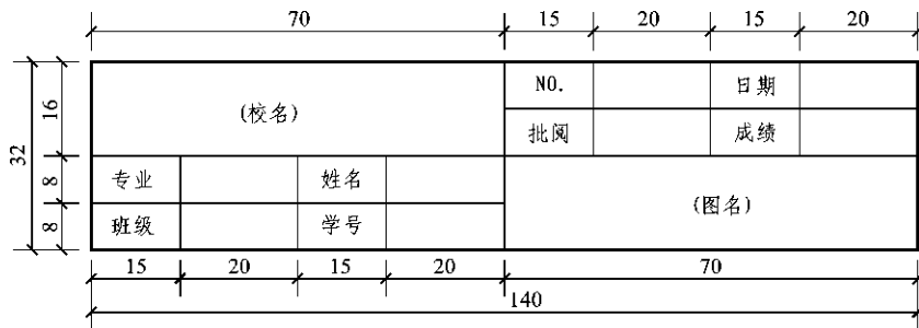
图 2-10 标题栏格式
