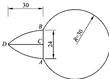
图 1-34 圆弧实例
