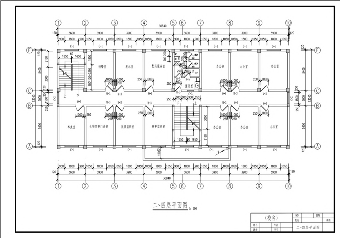
图 3-1 二~四层平面图
