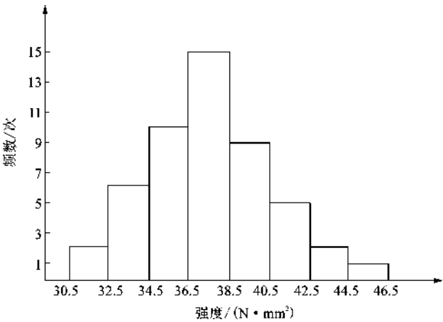
图 2-8 混凝土强度分布直方图
