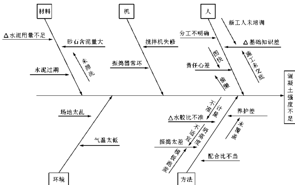
图 2-6 混凝土强度不合格因果分析图
