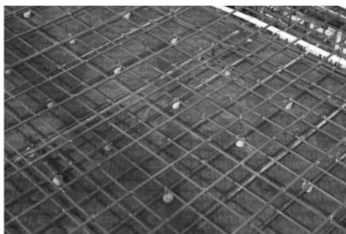
图 3-16 板钢筋设置数量足够的水泥砂浆保护层垫块
