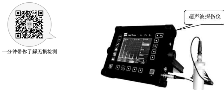
图 2-5 超声波探伤仪
