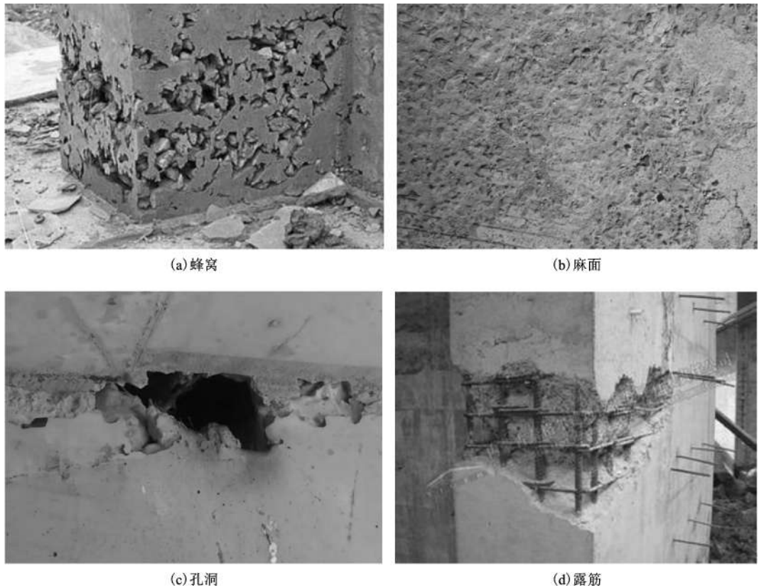
图 3-22 混凝土结构外观缺陷部分举例
