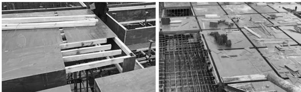
图 3-17 胶合木模板的安装
