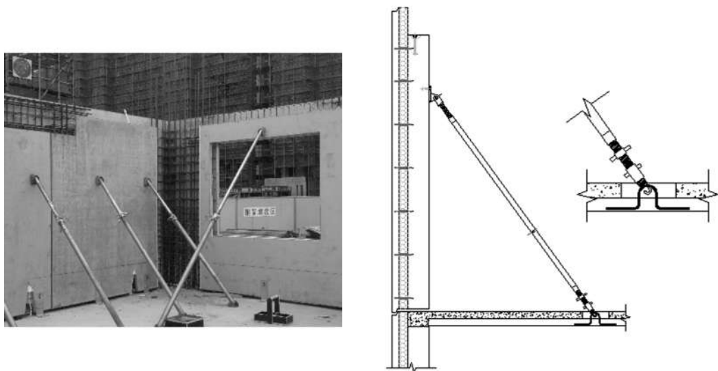
图 3-39 临时支撑
