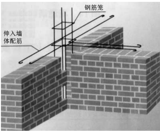
(a) 构造柱拉结筋锚入墙体
