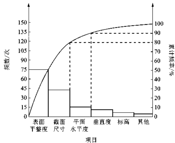
图 2-7 构件尺寸不合格点排列图
