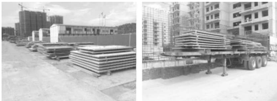
图 3-38 施工现场叠合楼板存放
