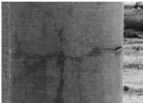
图 3-13 桩身断裂
