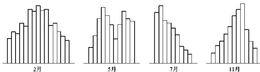
图 2-12 某工程混凝土预制板厚度直方图
