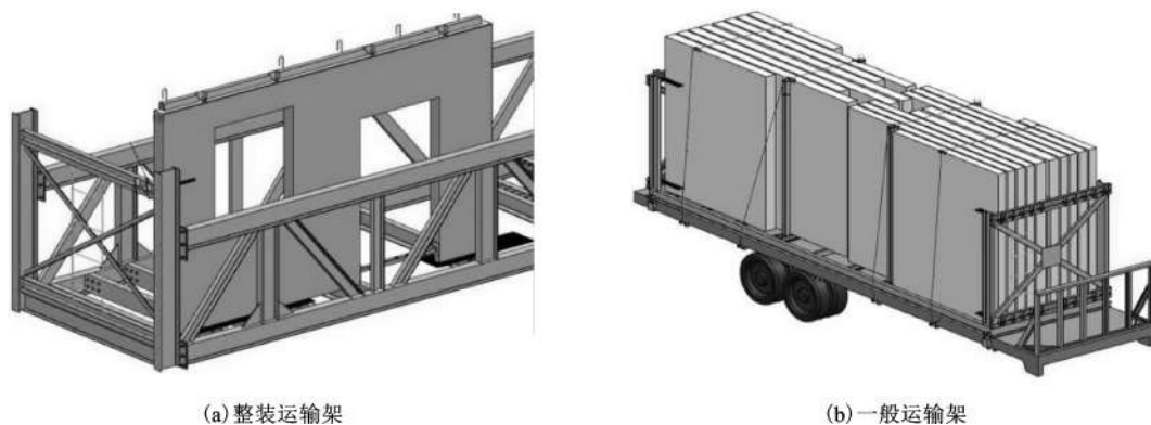
图 3-37 整装运输架和一般运输架
