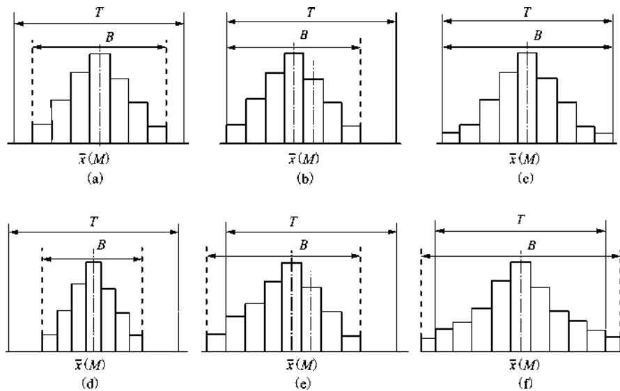
图 2-10 直方图与质量标准上、下限
