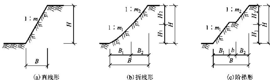
图 1-18 基坑边坡
