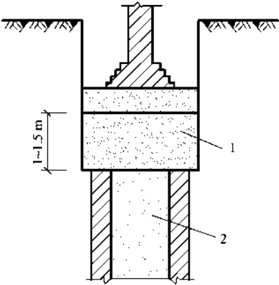
图 2-9 基槽下砖井处理方法
