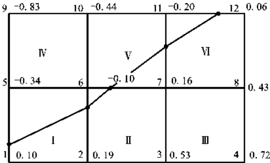
图 1-15 施工高度及零线位置
