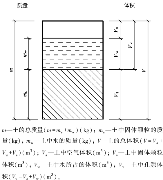
图 1-1 土的三相示意图
