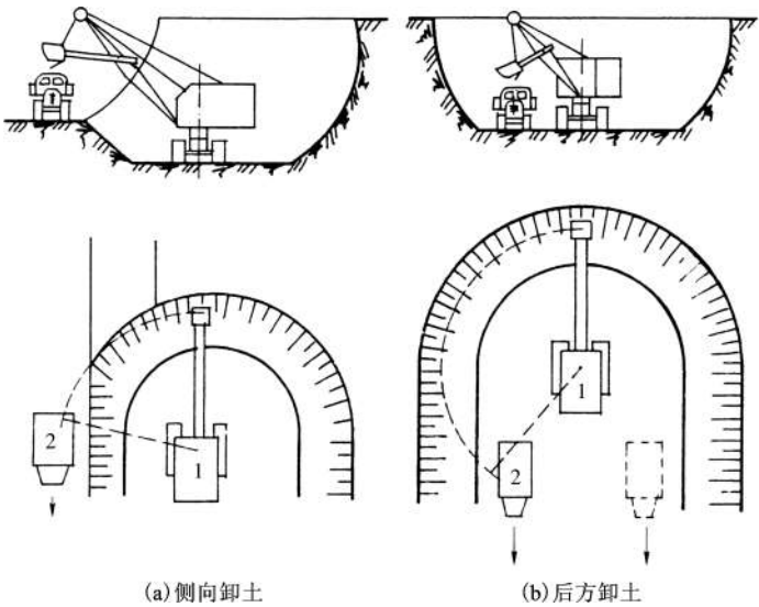
1—正铲挖土机；2—自卸汽车。
