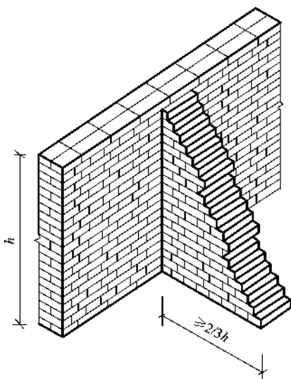
图 3-31 斜槎
