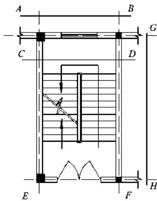
图 1-116 辅助线的位置
