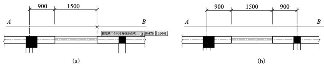
图 1-119 确定第二条尺寸界线及连续标注后的结果
