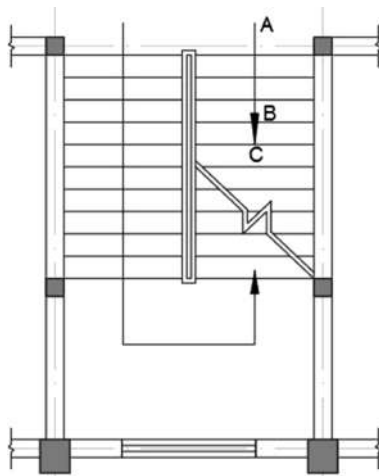
图 3-57 楼梯箭头标注
