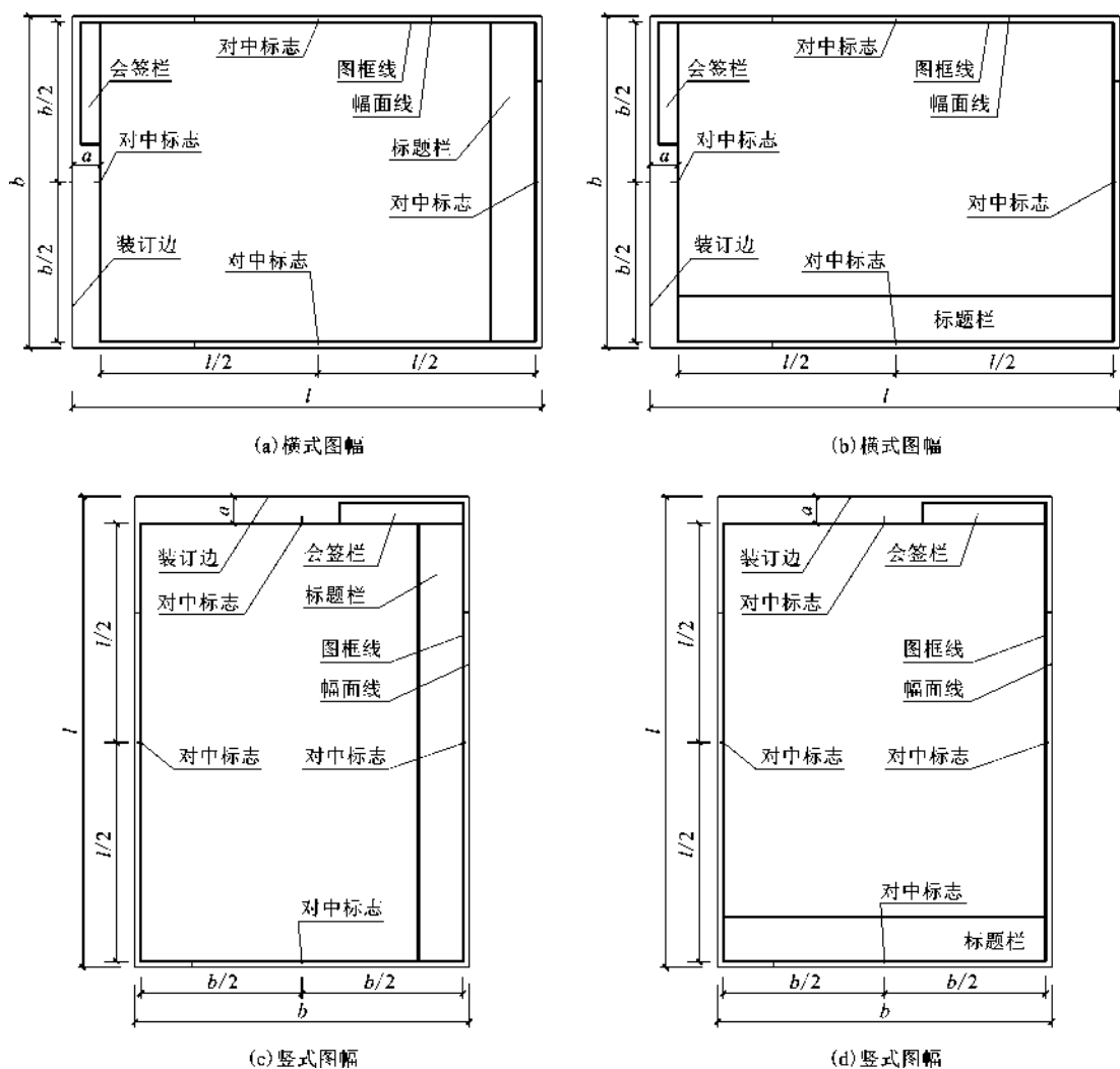
图 2-1 图纸格式
