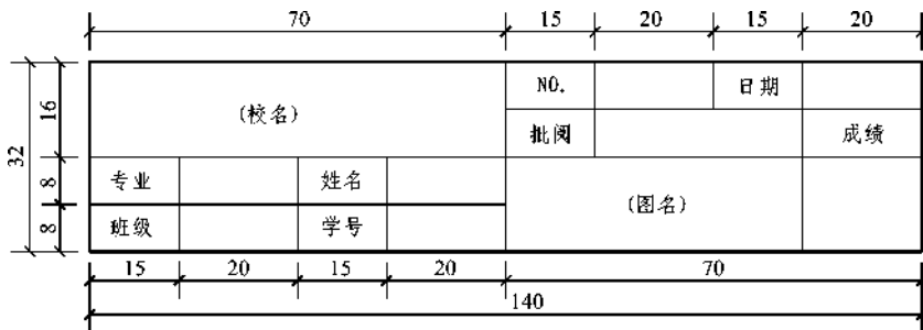
图 2-10 标题栏格式
