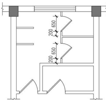
图 3-52 隔板门
