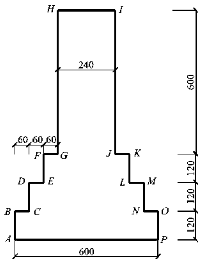
图 1-4 正交实例
