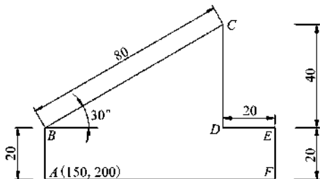
图 1-13 坐标输入实例
