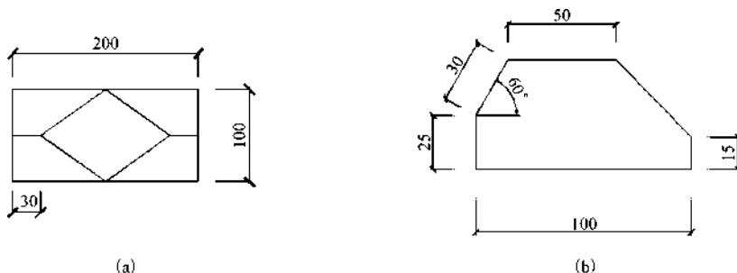
图 1-132 习题 1
