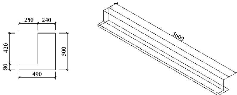
图 1-129 挑水屋檐
