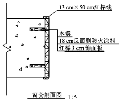
图 1-82 窗套剖面图说明文字
