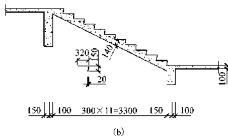
图 1-142 习题 11
