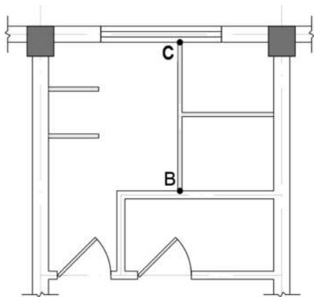
图 3-51 隔断与隔板
