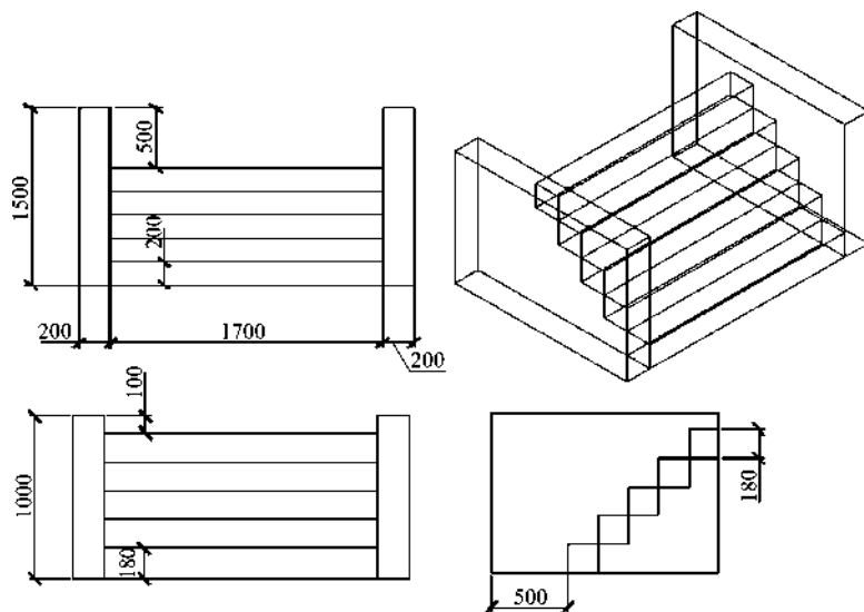
图 1-150 习题 19
