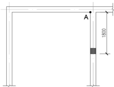
图 3-30 首个构造柱
