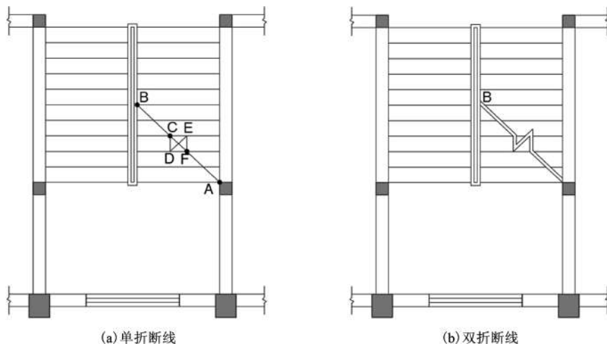
图 3-49 楼梯折断线
