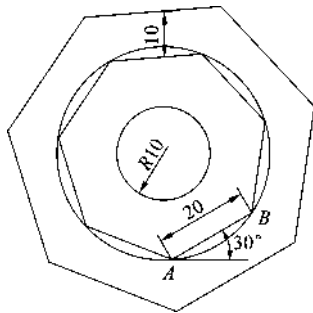
图 1-53 螺帽正投影图
