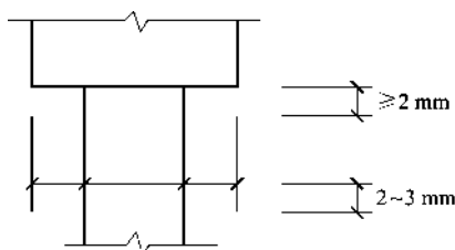
图 1-94 尺寸界线
