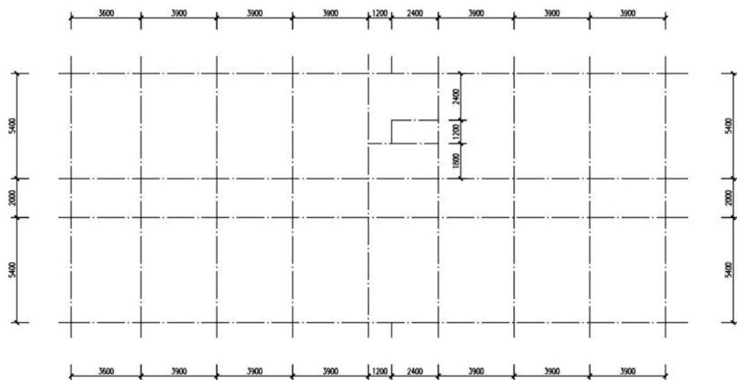
图 3-23 轴网尺寸标注
