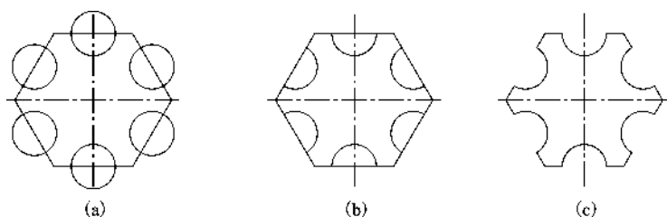
图 1-44 修剪实例
