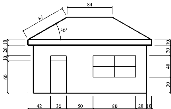
图 1-26 平房立面图
