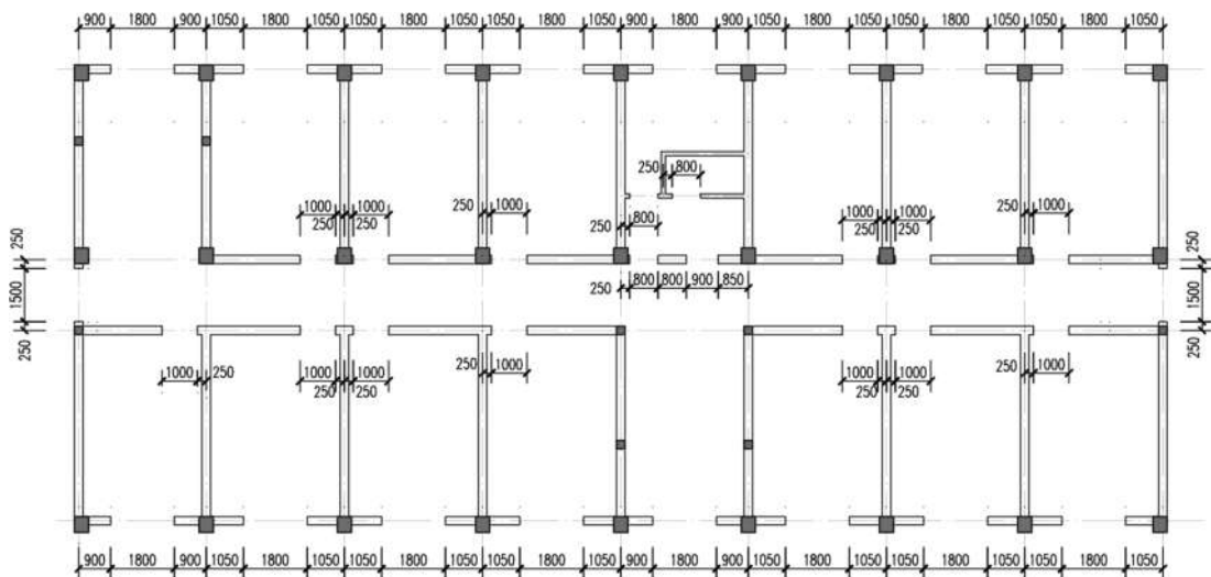
图 3-37 门窗洞口
