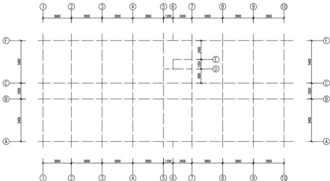
图 3-25 轴号标注
