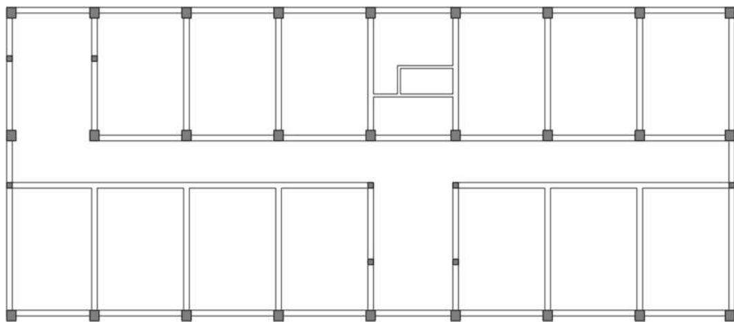
图 3-34 柱网
