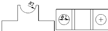
图 1-110 半径、直径与圆心标注
