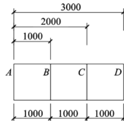
图 1-108 基线标注
