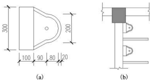
图 3-55 小便器
