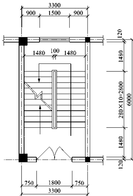
图 1-113 楼梯详图尺寸
