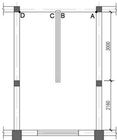
图 3-46 楼梯梯井
