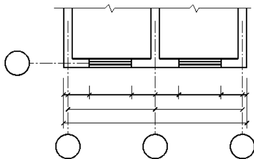
图 1-95 尺寸的排列
