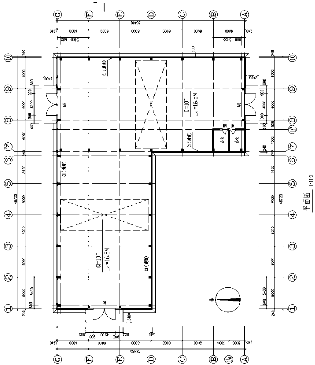
图 3-65 单层厂房平面图
