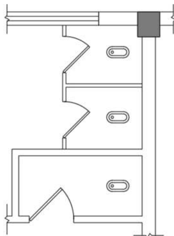
图 3-54 蹲便器
