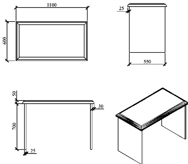
图 1-149 习题 18
