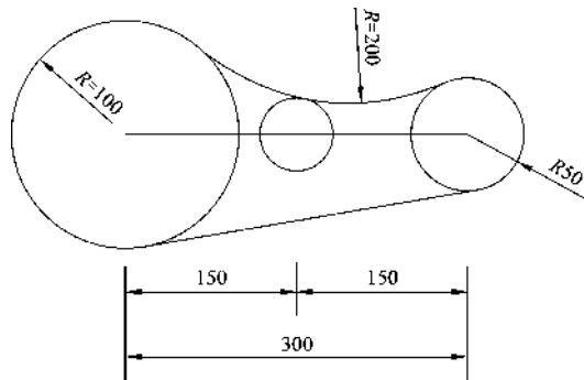
图 1-50 皮带传动图
