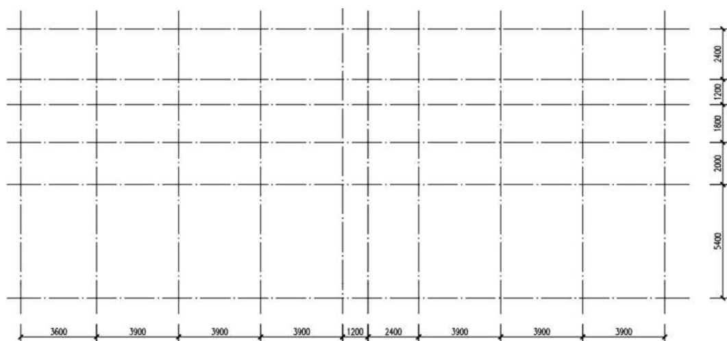
图 3-10 轴网
