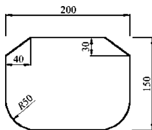
图 1-49 倒角实例
