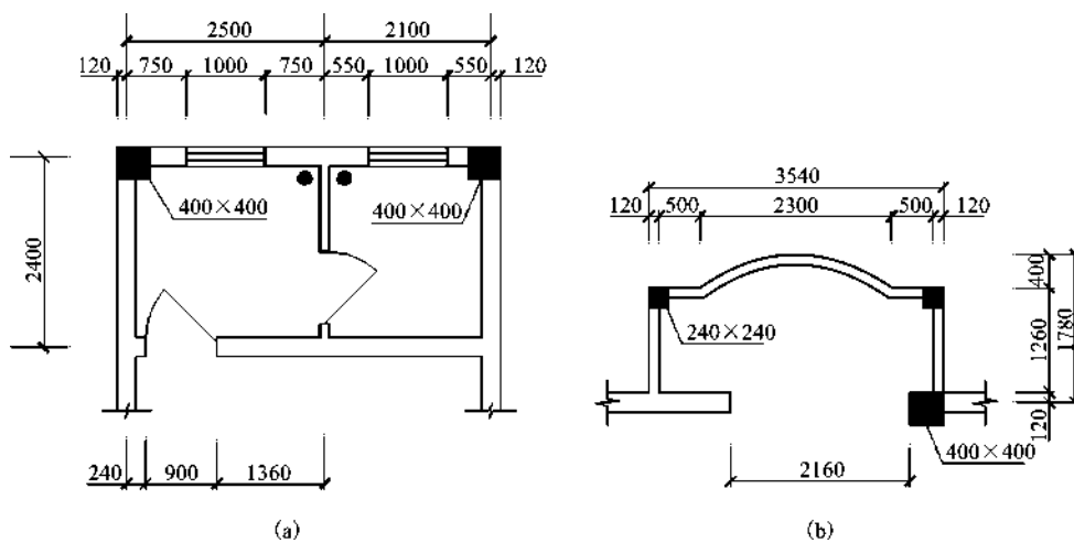
图 1-146 习题 15
