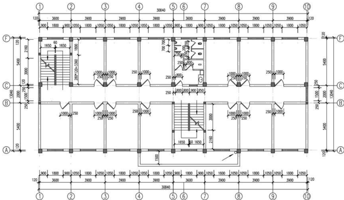
图 3-61 尺寸标注
