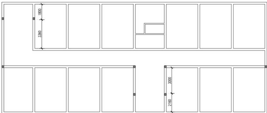
图 3-32 所有构造柱
