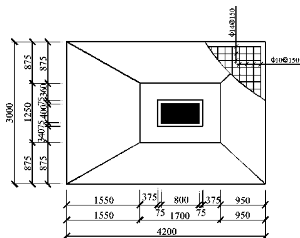
图 1-145 习题 14
