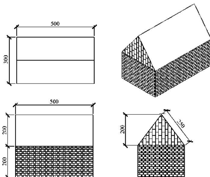
图 1-148 习题 17
