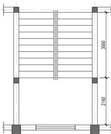
图 3-48 楼梯梯段线
