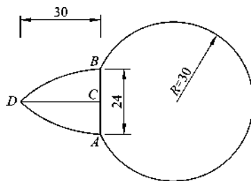
图 1-34 圆弧实例
