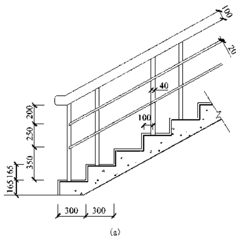
图 1-142 习题 11
