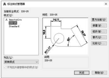
图 1-97 “标注样式管理器”对话框
