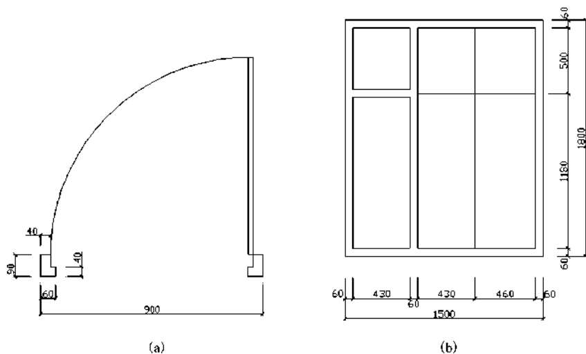
图 1-133 习题 2
