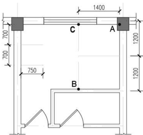
图 3-50 隔断与隔板定位线
