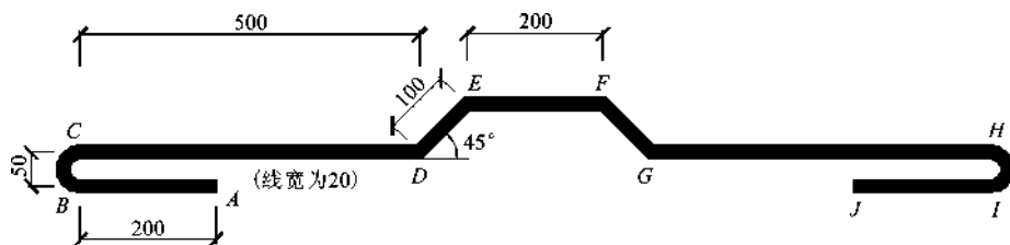
图 1-18 绘制钢筋
