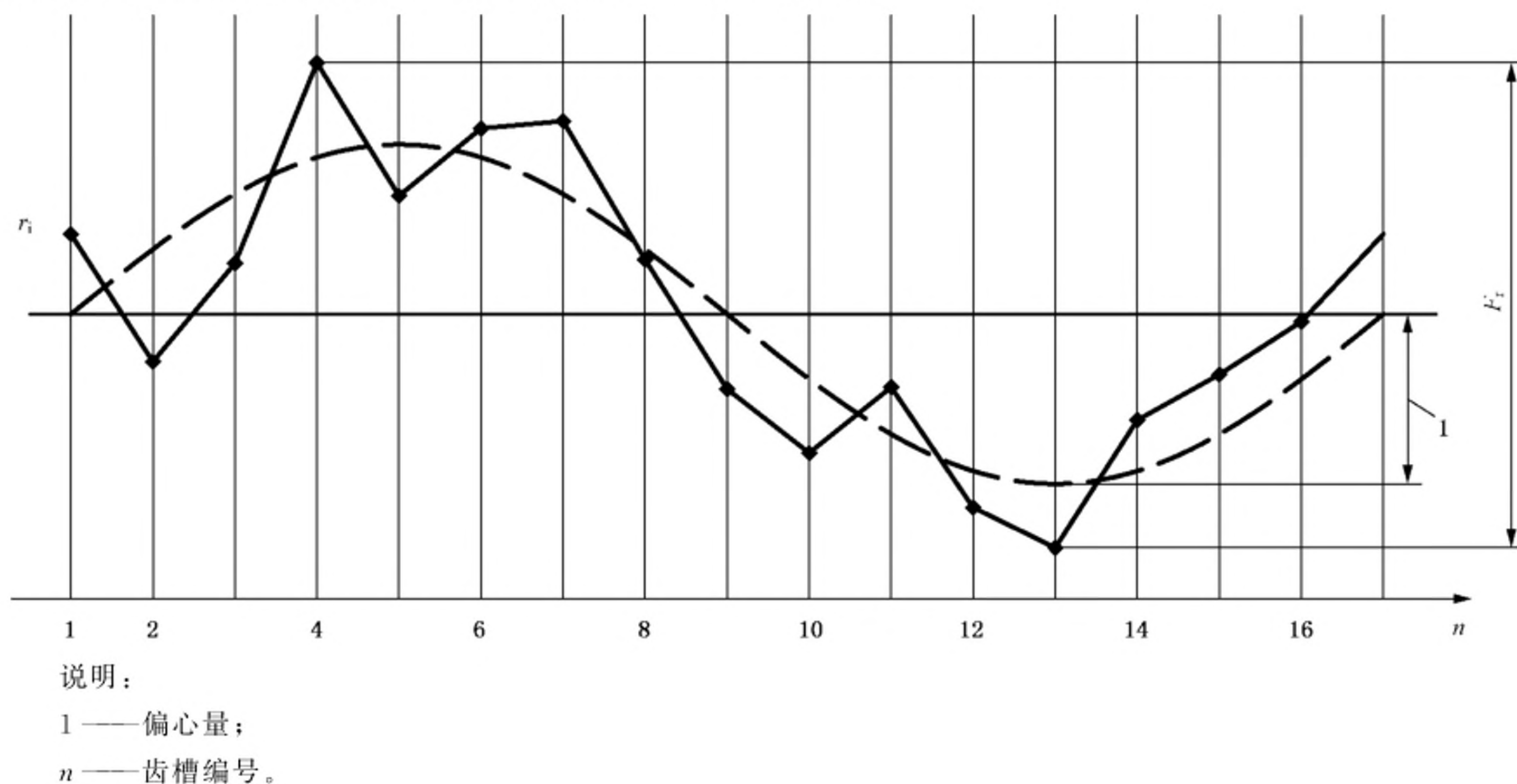
图 E.1 有 16 个齿齿轮的径向跳动
