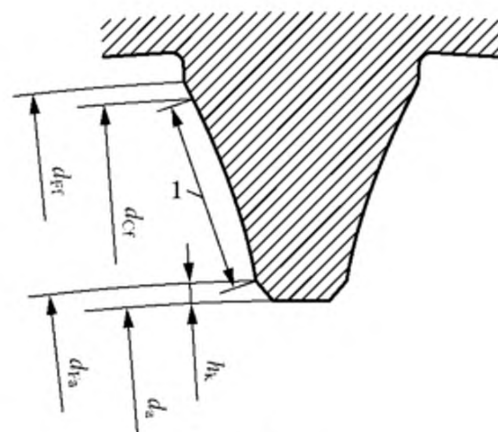
b) 内齿轮
