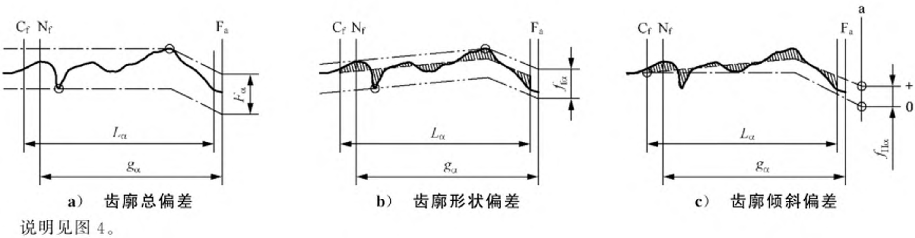
图 7 齿顶修缘的齿廓偏差
