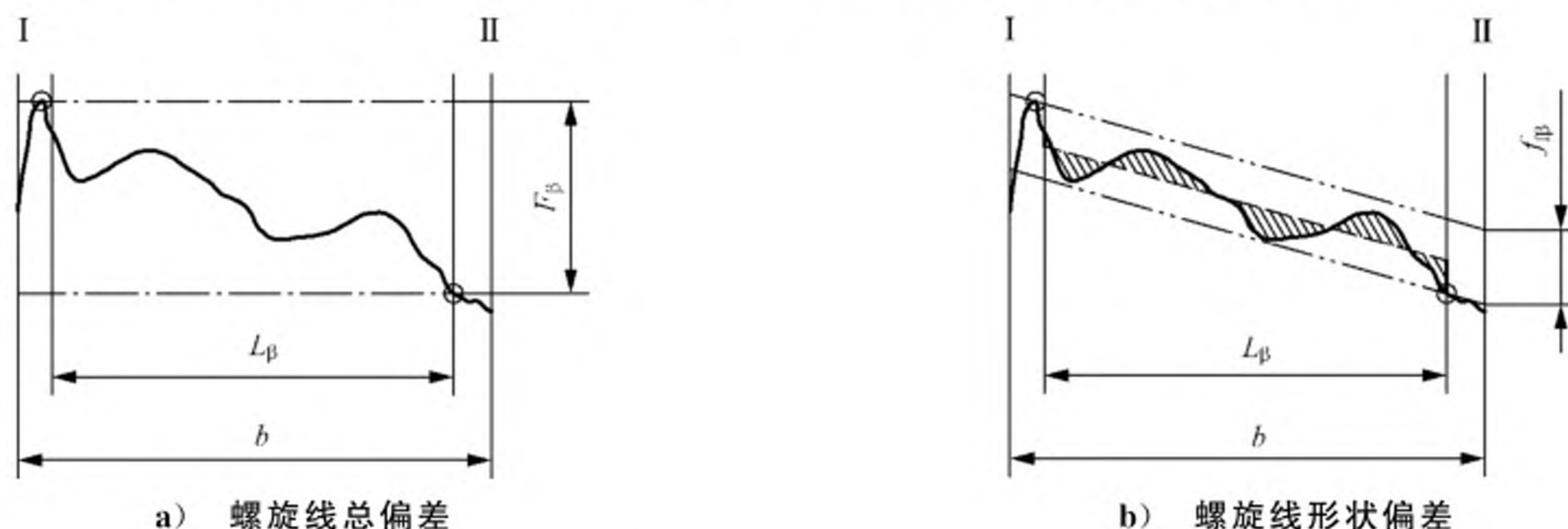
图 15 螺旋线偏差的评价
