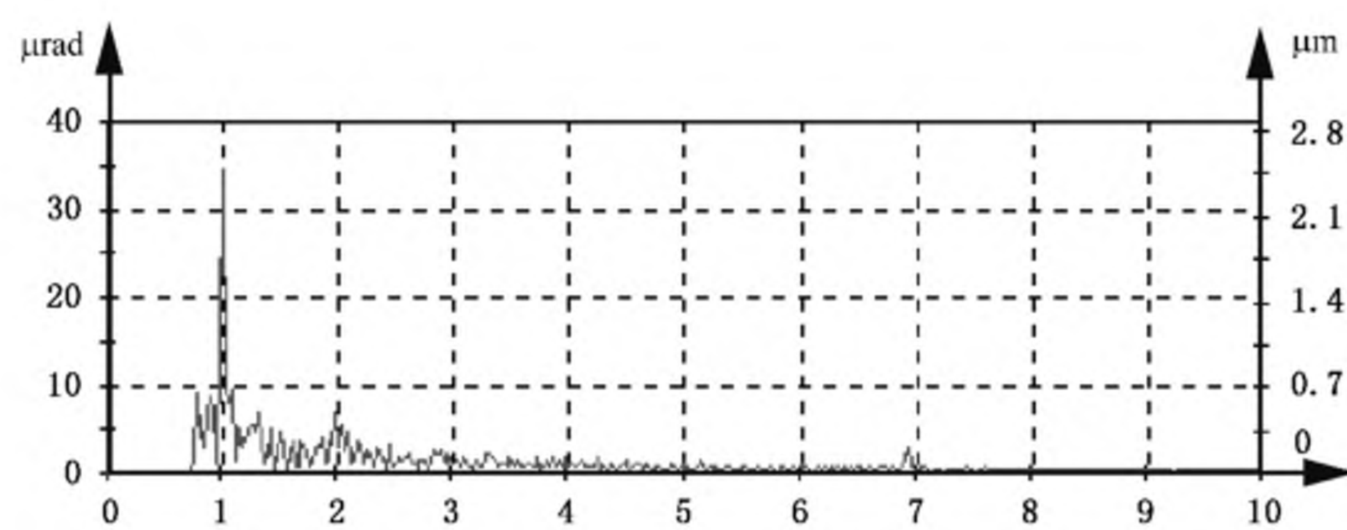
a) 啮合频率的阶次-线性幅值
