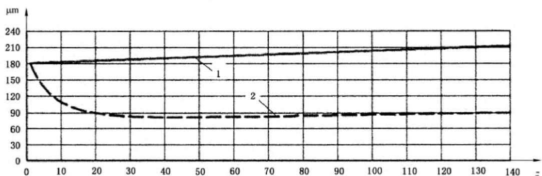
c) 公差等级为 R50 的径向综合公差
