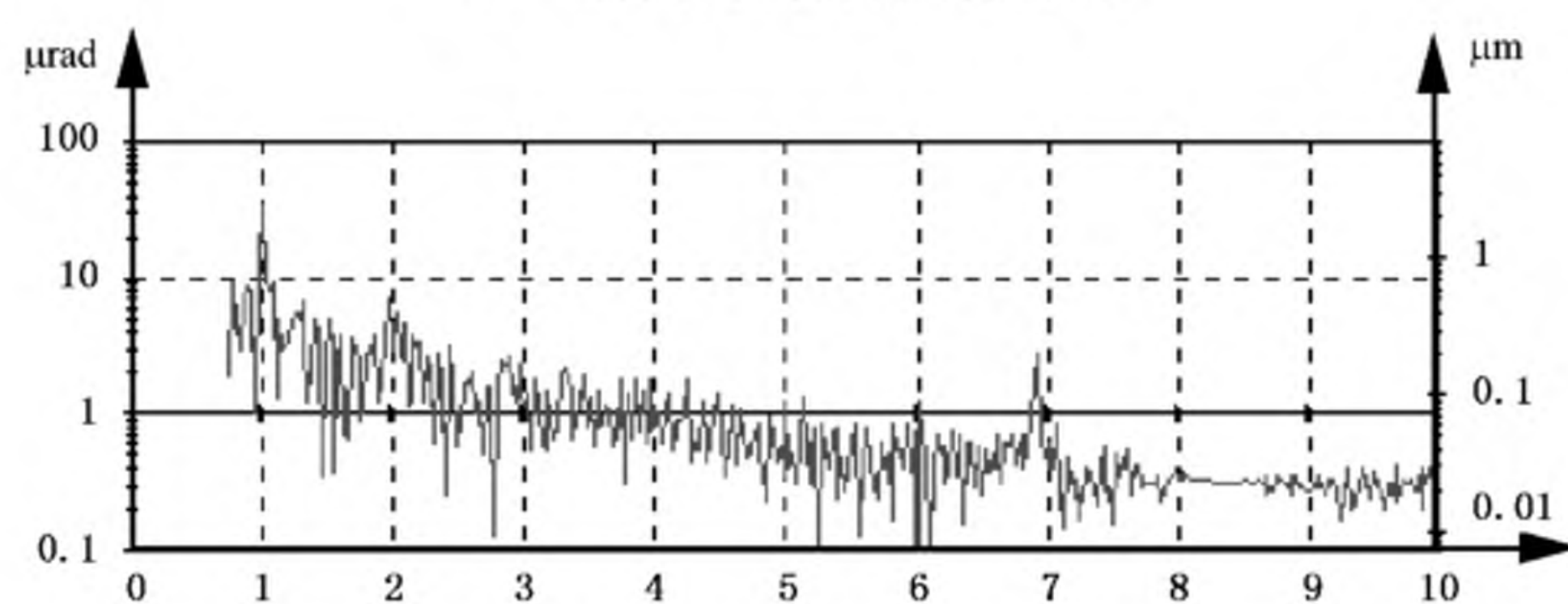
b) 啮合频率的阶次-对数幅值
