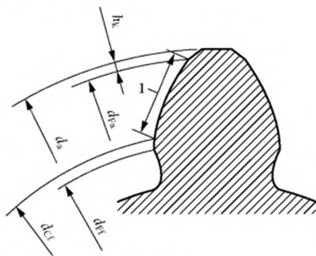
a) 外齿轮
