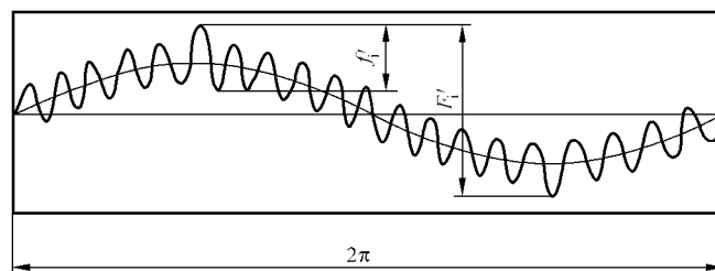
图3 蜗轮旋转时单面啮合偏差 F'_{i1} 和单面一齿啮合偏差 f'_i
