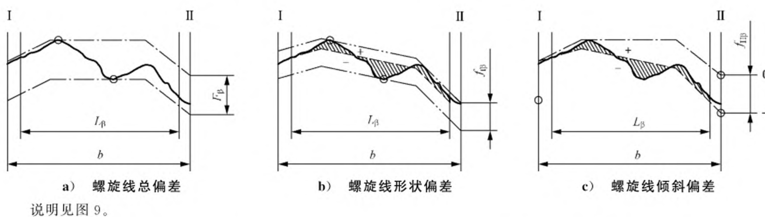
图 12 螺旋线齿端修薄的螺旋线偏差
