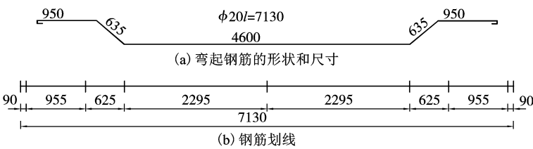
图 1 弯起钢筋的划线
