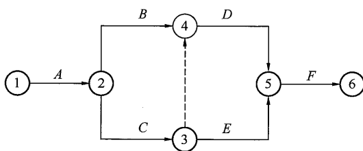
图 4.1.1 双代号网络图
