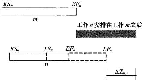
图 12 m, n 两项工作的排序
