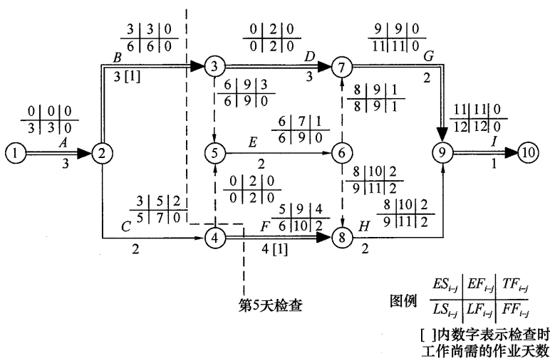
图 14 双代号网络计划实施检查实例
