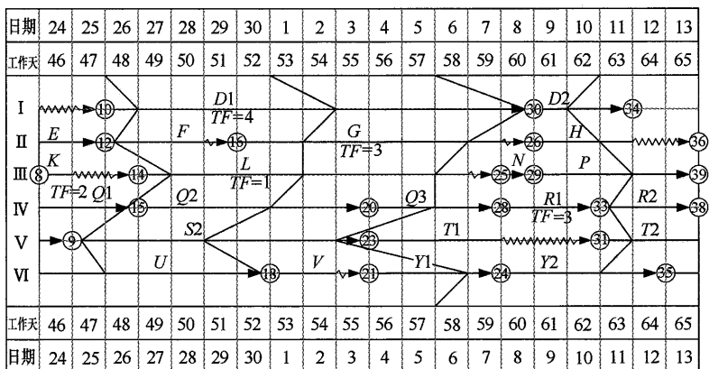
图 13 实际进度前锋线示例
