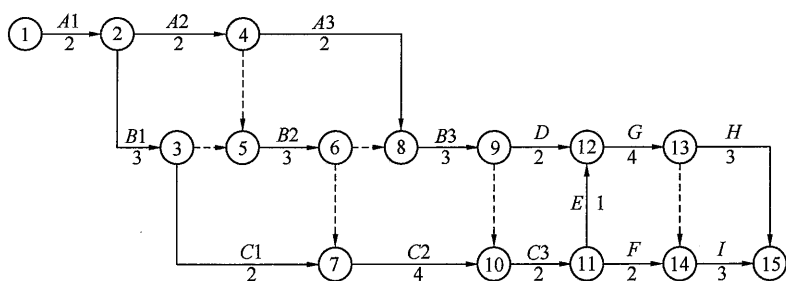
图 5 双代号网络计划
