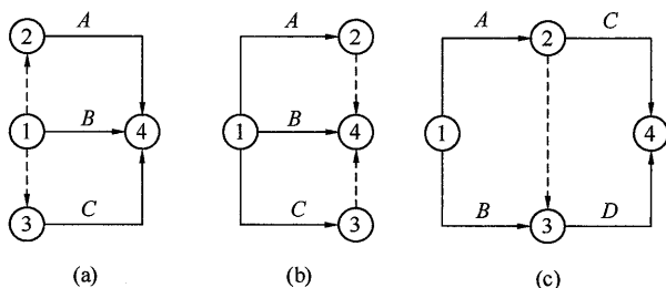
图 2 双代号网络图中虚箭线的应用示意图
