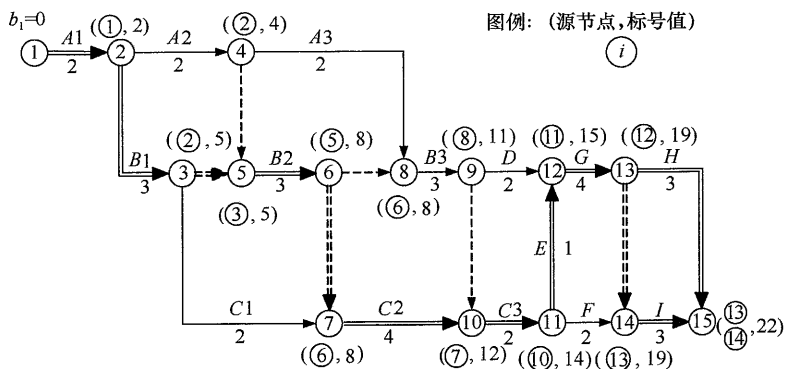
图 11 标号法确定关键工作和关键线路
