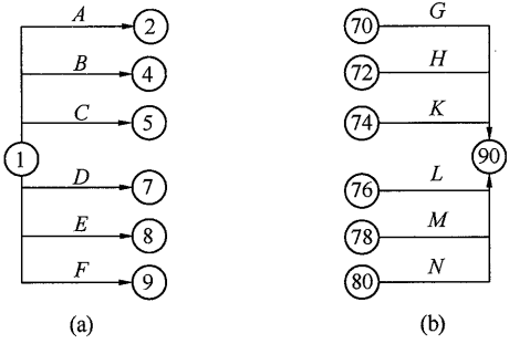
图 3 母线法绘制
