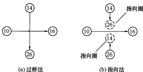
图 4 箭线交叉的表示方法
