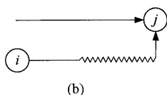
图9 工作有自由时差时波形线画法
