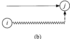
图10 虚工作有自由时差时波形线画法
