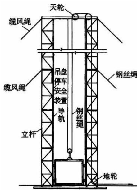
龙门架的基本构造形式
