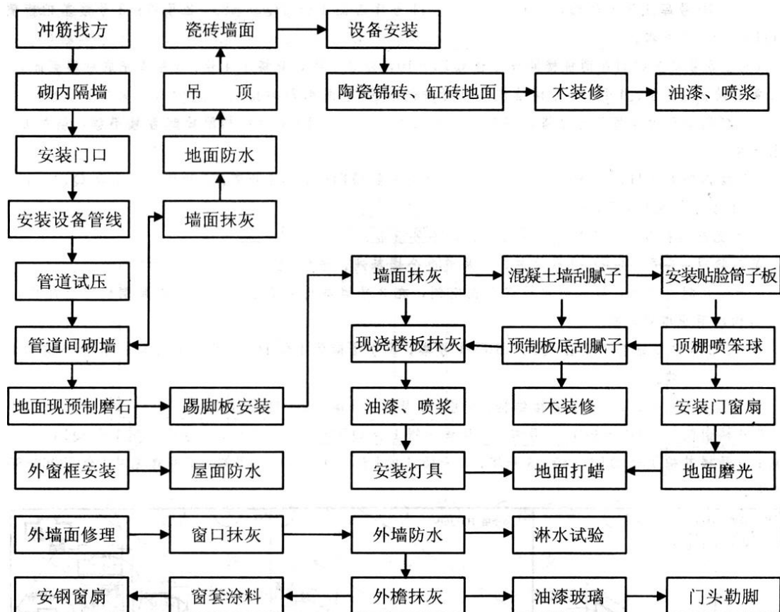
图 6-29 装修工程工艺流程图
