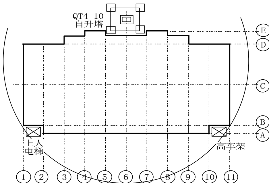
图 6-31 住宅结构阶段 QT4-10 自升塔布置示意图
