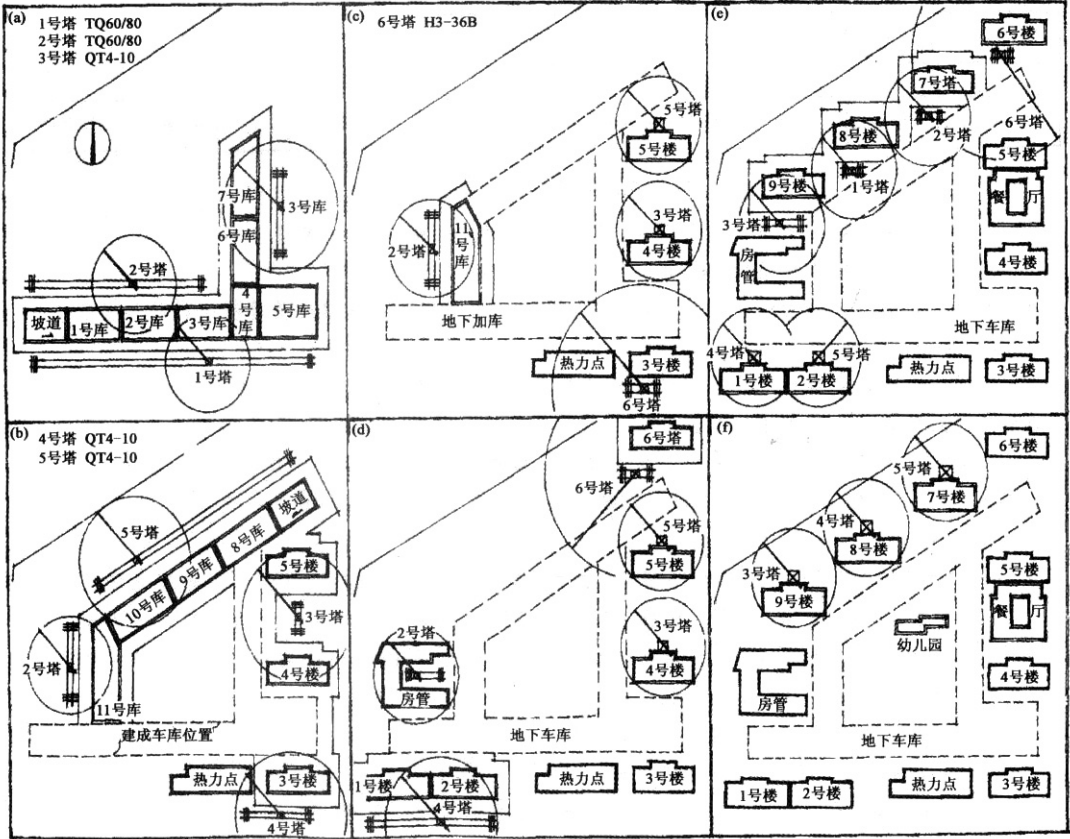
图 6-30 塔式起重机布置示意图
