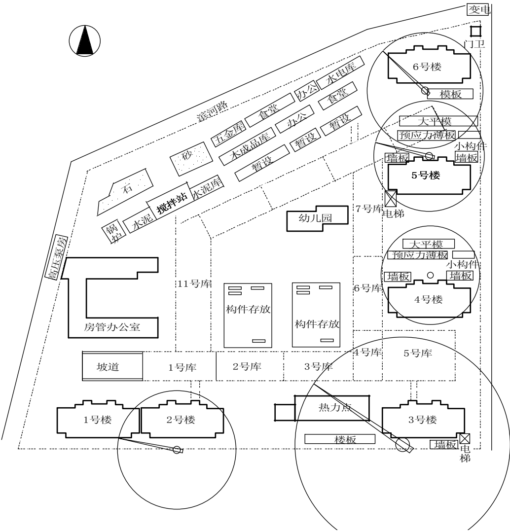
图 6-28 施工总平面布置图
