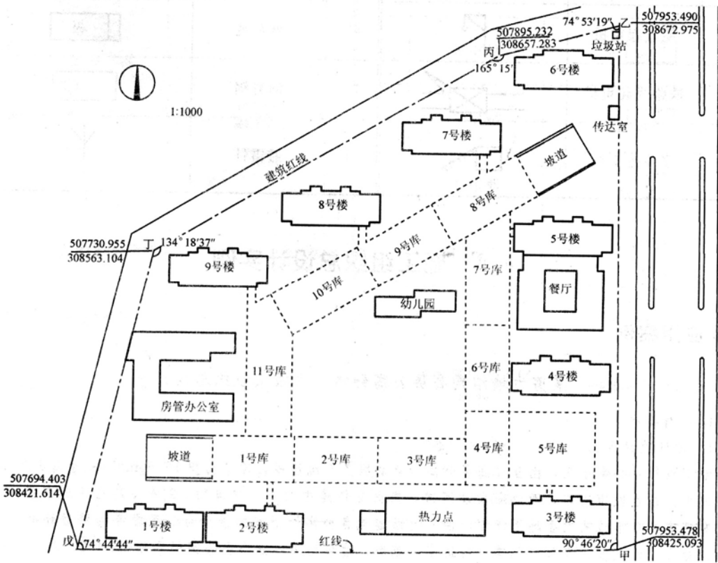
图 6-25 住宅小区平面图
