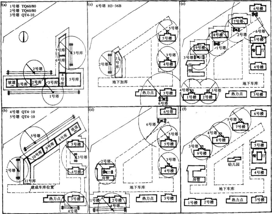
图 塔式起重机布置示意图
