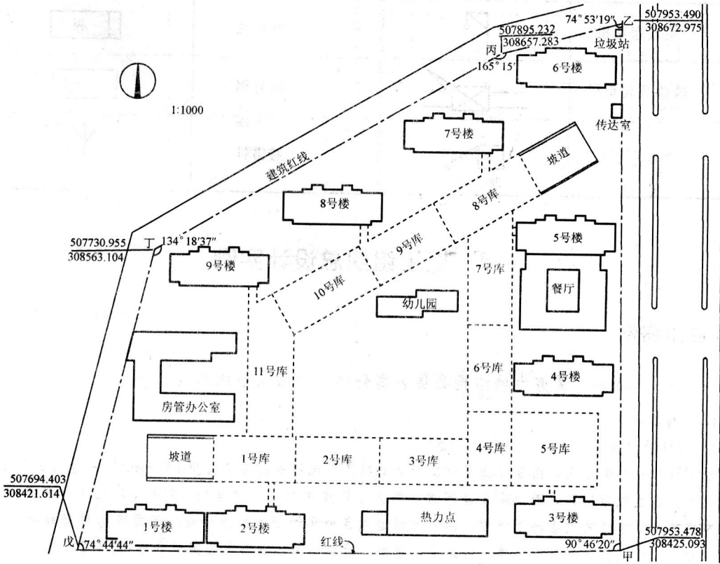
图1 住宅小区平面图
