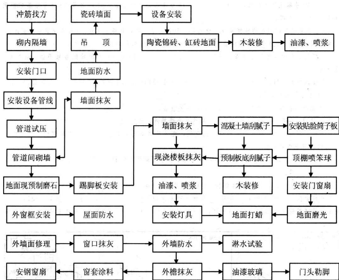
图 装修工程工艺流程图
