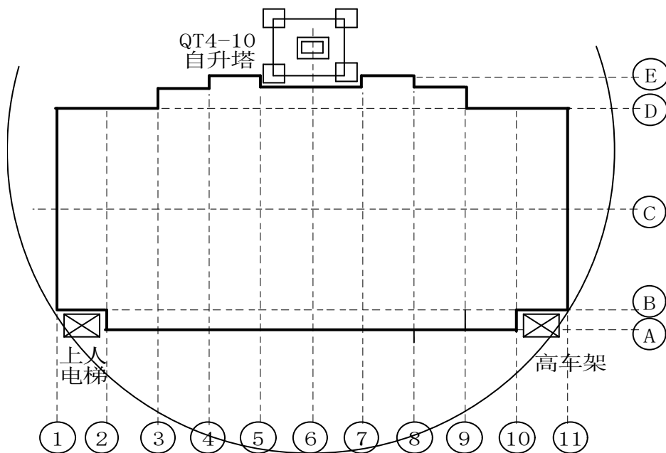
图 住宅结构阶段 QT4-10 自升塔布置示意图
