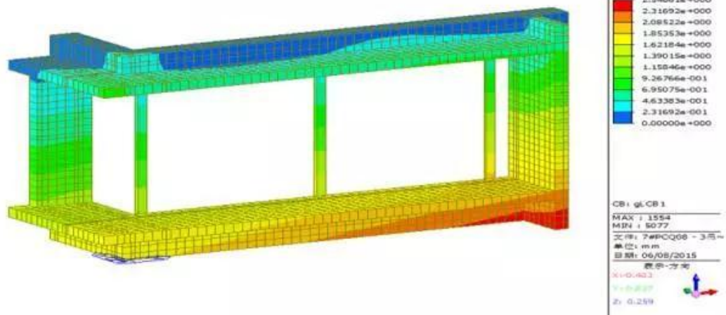
▲ 力学验算
