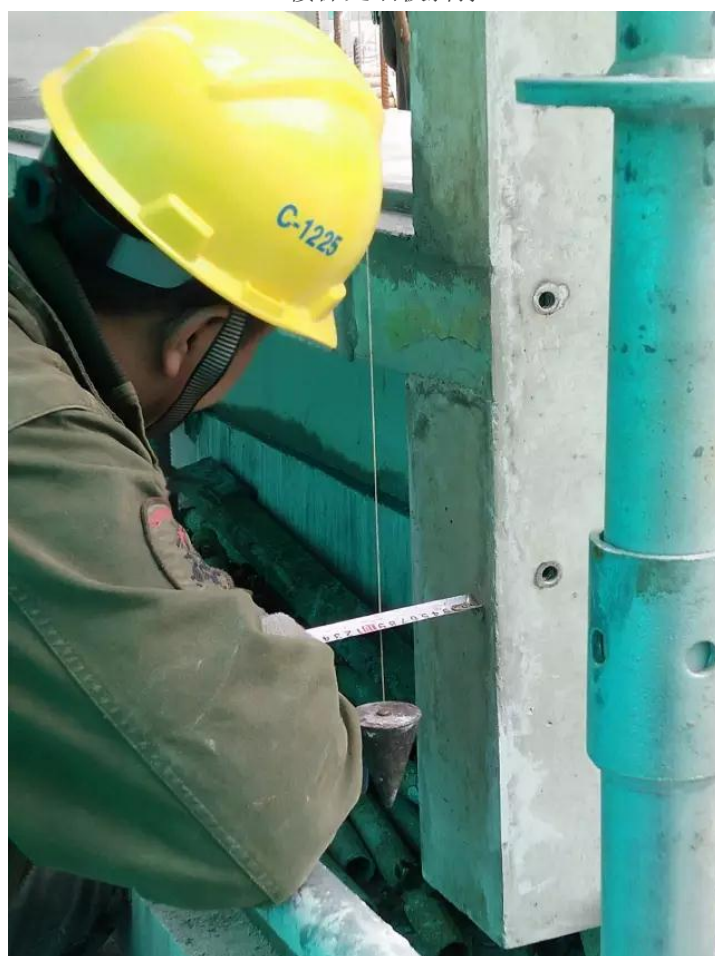
▲ 构件测垂直
