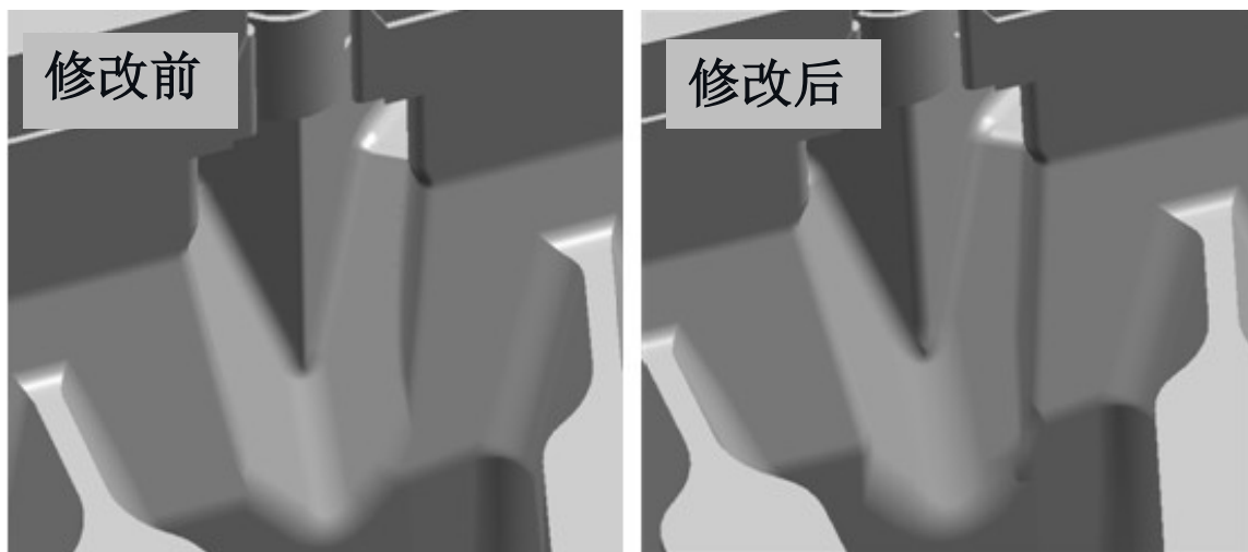
模具引流斜槽优化前后对比图
