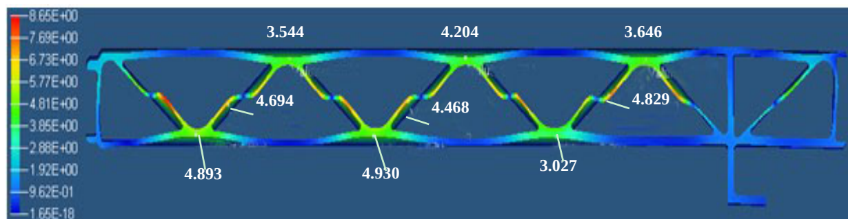
初始设计方案模拟的挤出型材变形分布图
