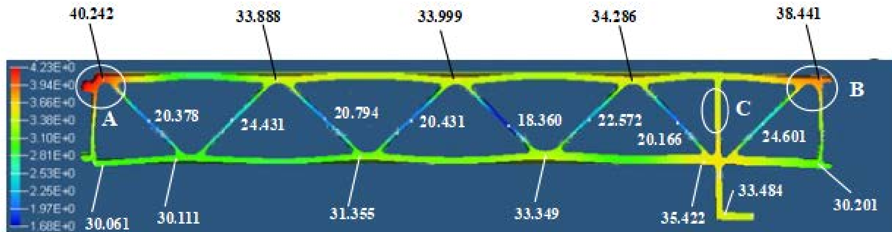
第一次优化后模拟的挤出型材速度分布图（单位：mm/s）
