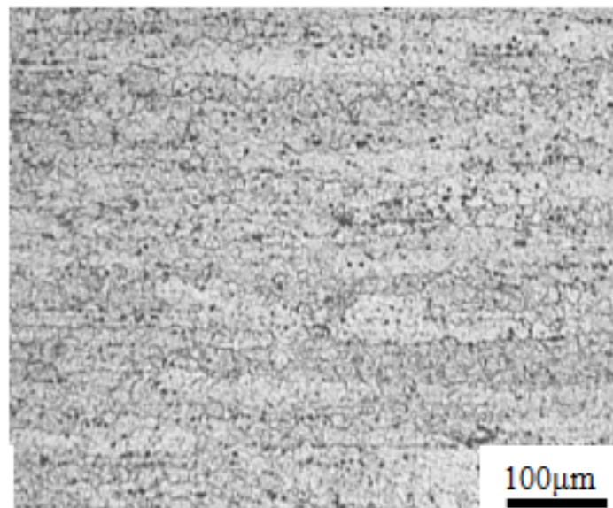
挤压方向纵断面金相组织
