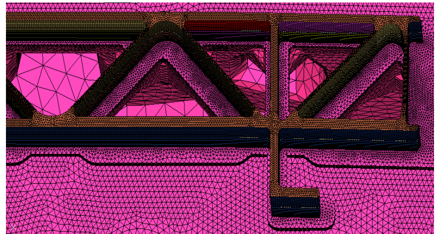
计算机仿真模拟模型
