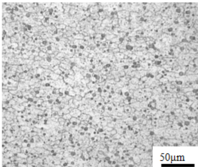
挤压方向横断面金相组织
