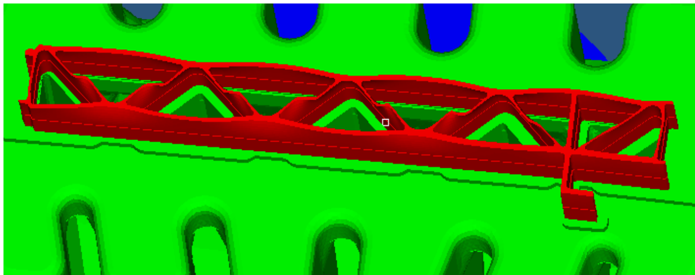
初始设计方案模拟的挤出型材图
