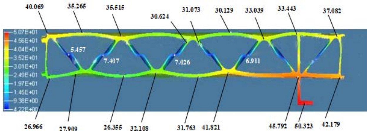
初始设计方案模拟的挤出料头速度分布图
