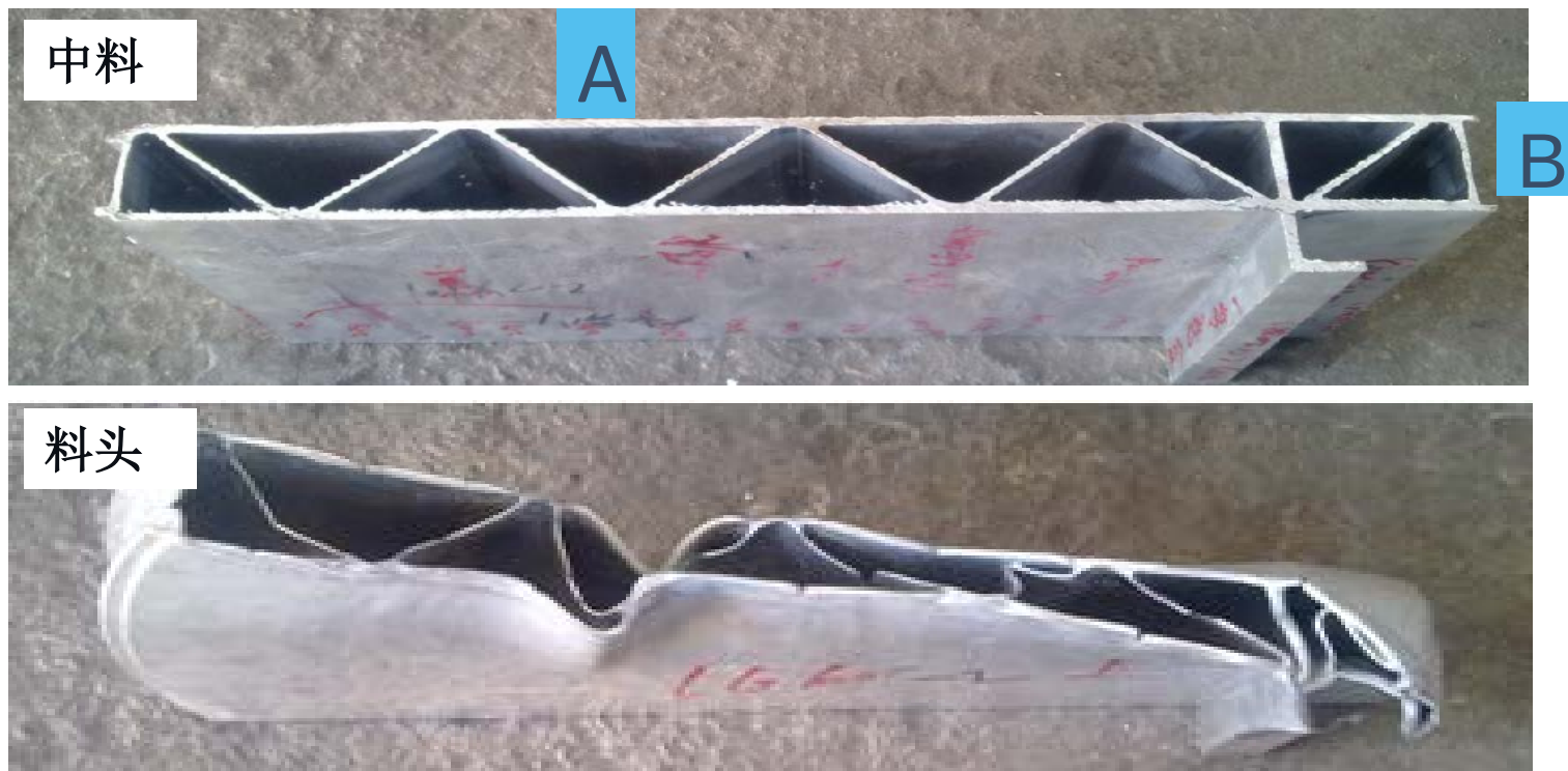
第一次试模挤出型材实物图
