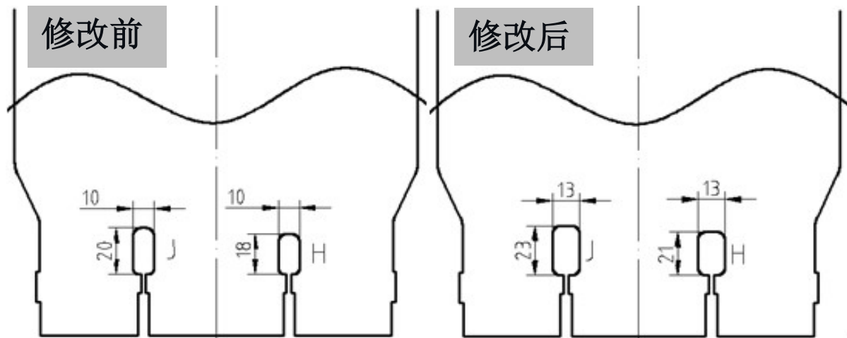
模具引流通孔第一次优化前后对比图
