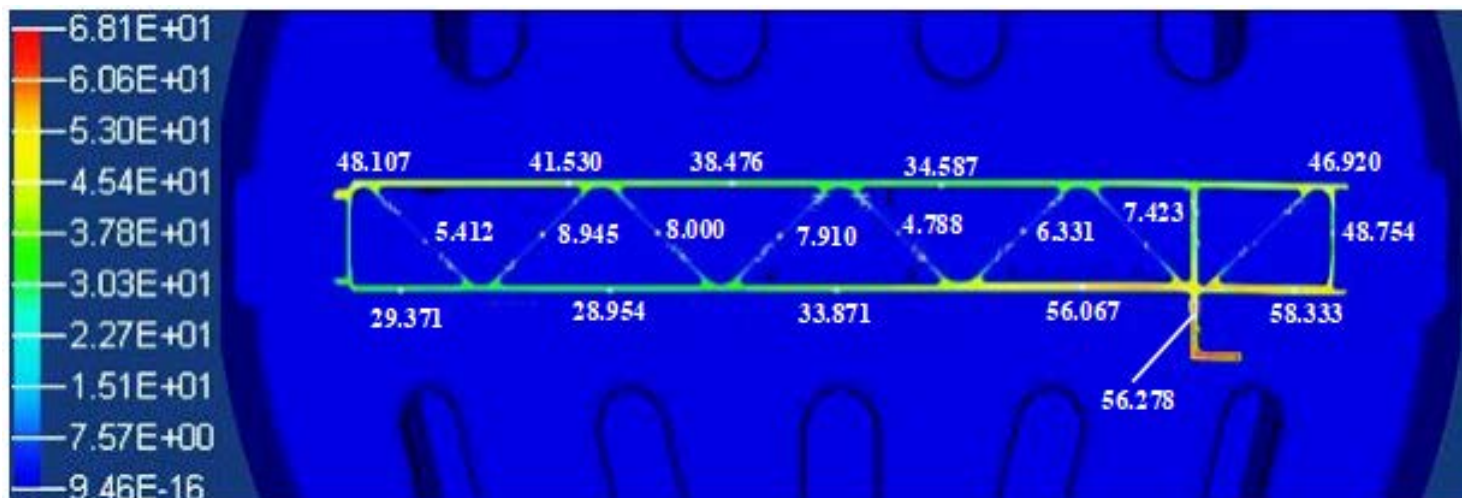
初始设计方案模拟的模孔金属流速分布图
