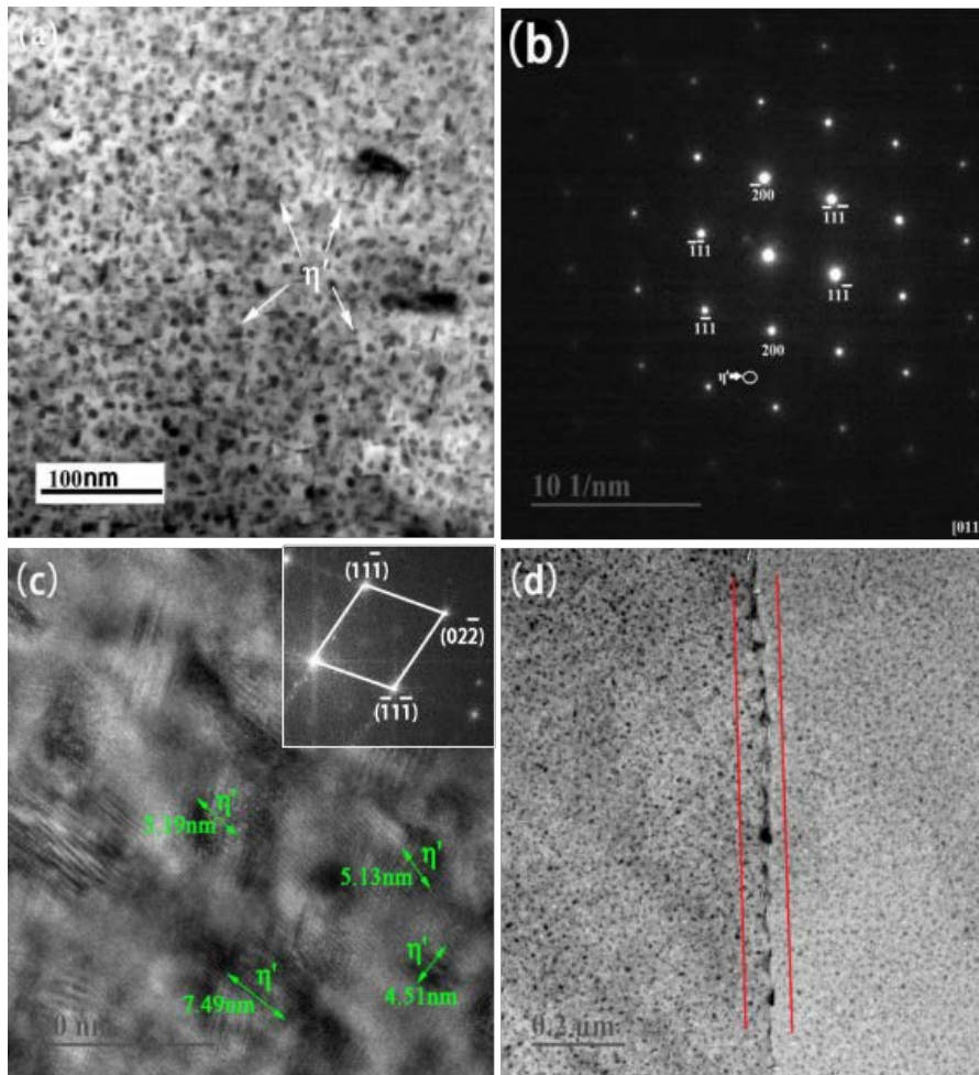
7055铝合金的TEM微观组织（ \langle 011 \rangle 晶带轴入射）（TEM） (a) 沉淀相明场像图片；(b) 与图 (a) 对应的衍射斑图像； (c) 沉淀相高分辨图像；(d) 晶界明场像图片
