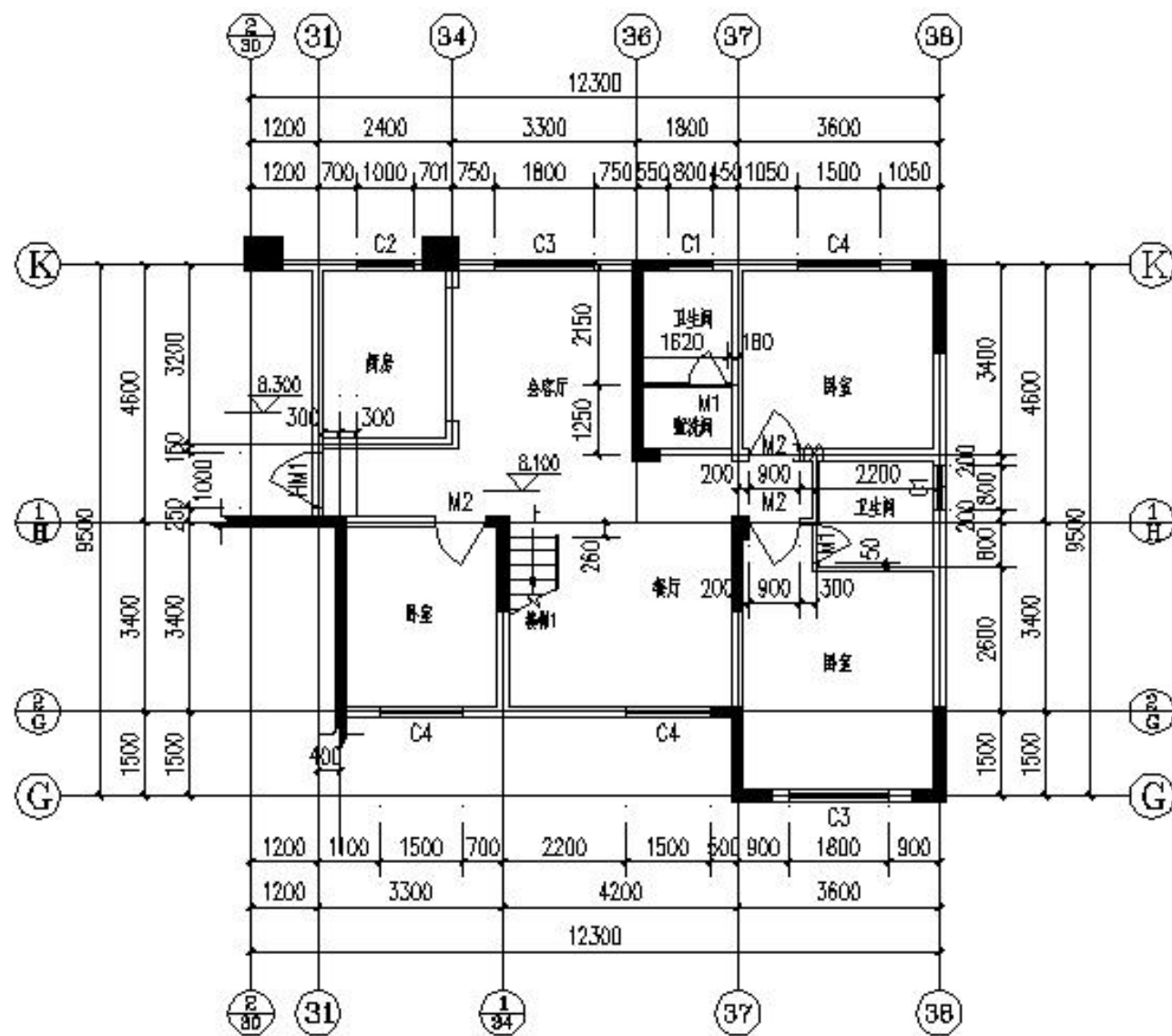
三层局部变更图 1:100
