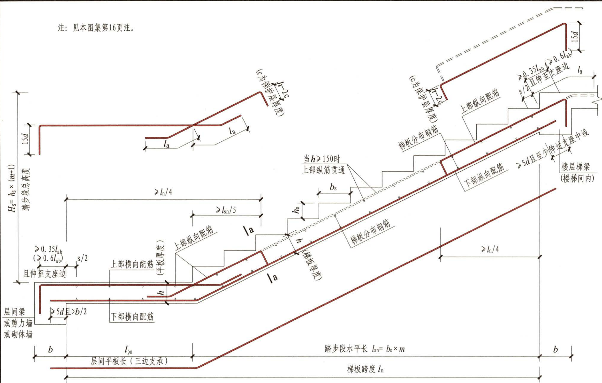
GT型楼梯梯板钢筋构造(2-2)
