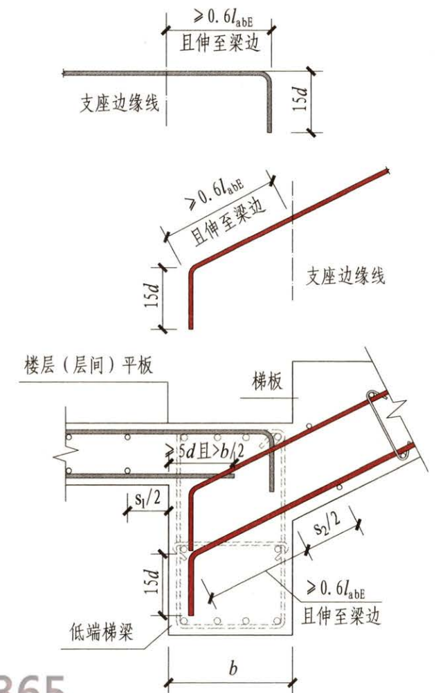
ATc低端梯梁处、梯板上、下部纵筋弯折段错开
