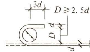
(a) 光圆钢筋末端180°弯钩
