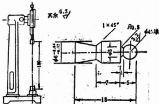
图 12.0.2-1 收缩仪 (mm) 1—千分表 2—支架
