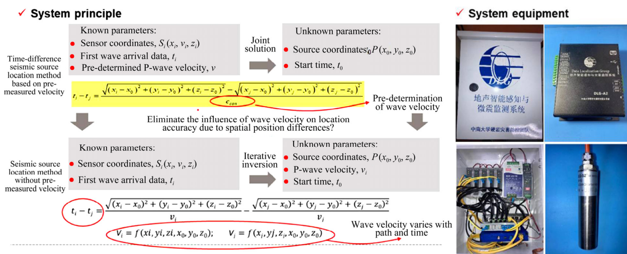
图 6 微震数据采集系统原理及设备 [37]
