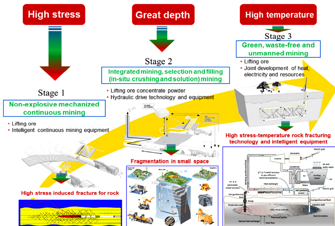
图2 深部开采三步走战略 [24-25]
