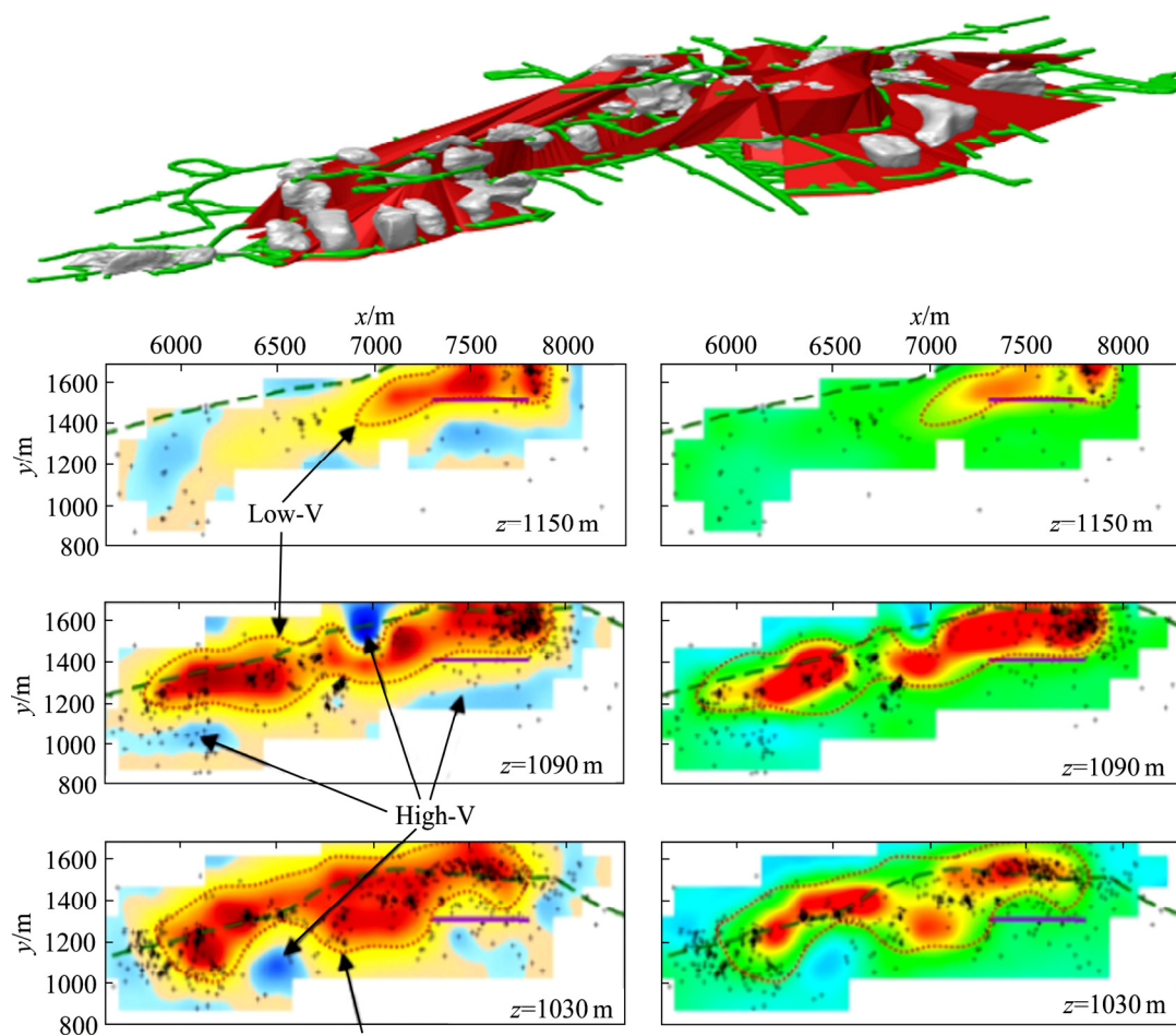
图 4 三维波速场层析精准反演采场的时移地震层析成像 [29]
