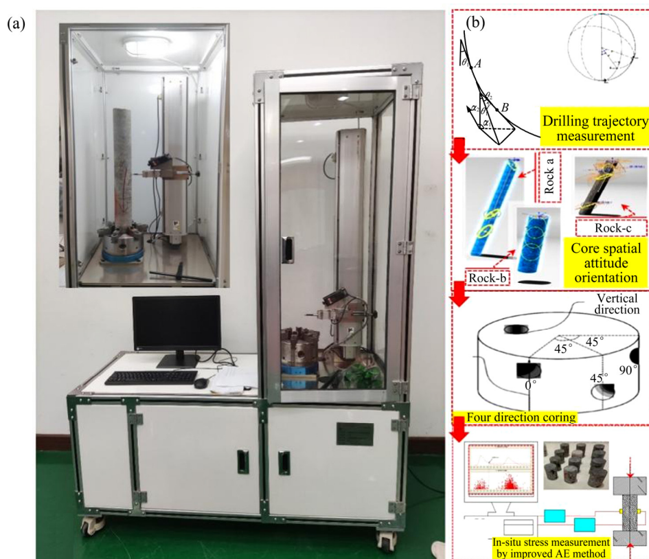
图5 岩芯地表重定位测量实验设备和基于岩芯地表重定位技术的声发射地应力测量方法作业流程 [33-35]
