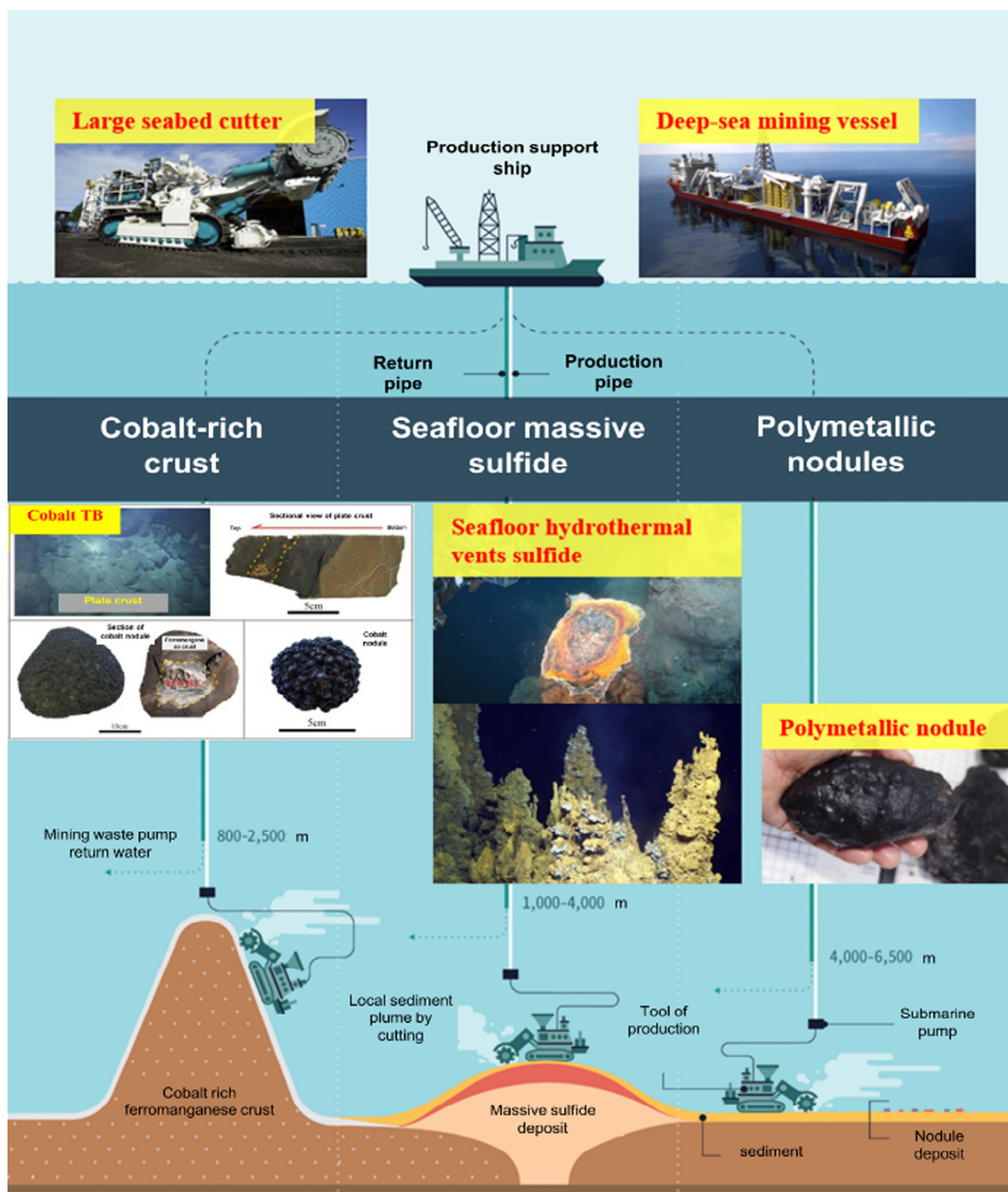
图 8 深海采矿作业 [47]
